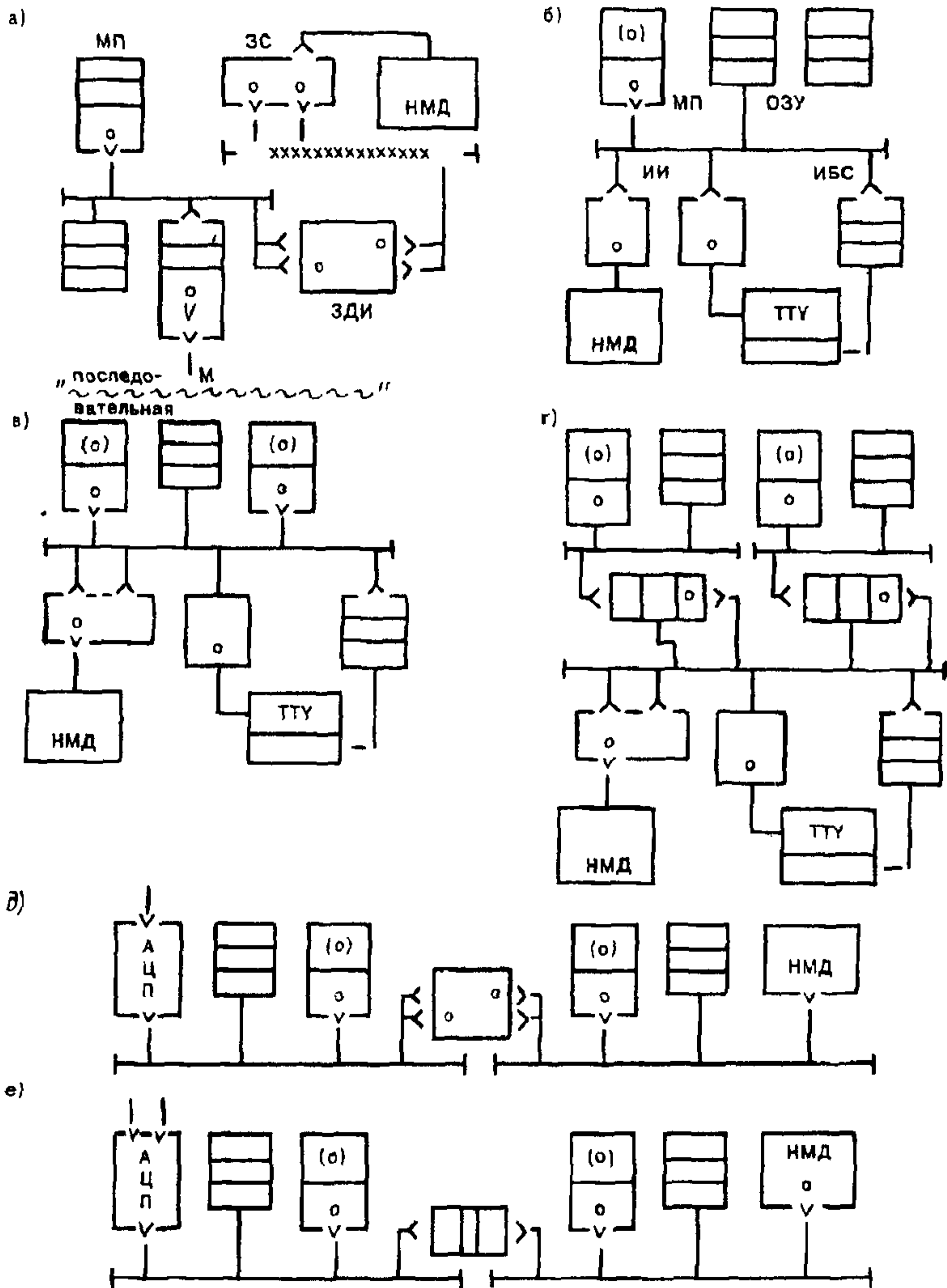
а) одноплатная микроЭВМ, подключенная через кабельную магистраль МСИ к НМД; б) персональная ЭВМ. ТТУ; в) двухпроцессорная микроЭВМ; г) вычислительная система с локальными подсистемами обработки данных; д) связь двух микроЭВМ через ЗДИ (прямой доступ в память); е) связь двух микроЭВМ через ИС (общее ОЗУ)
