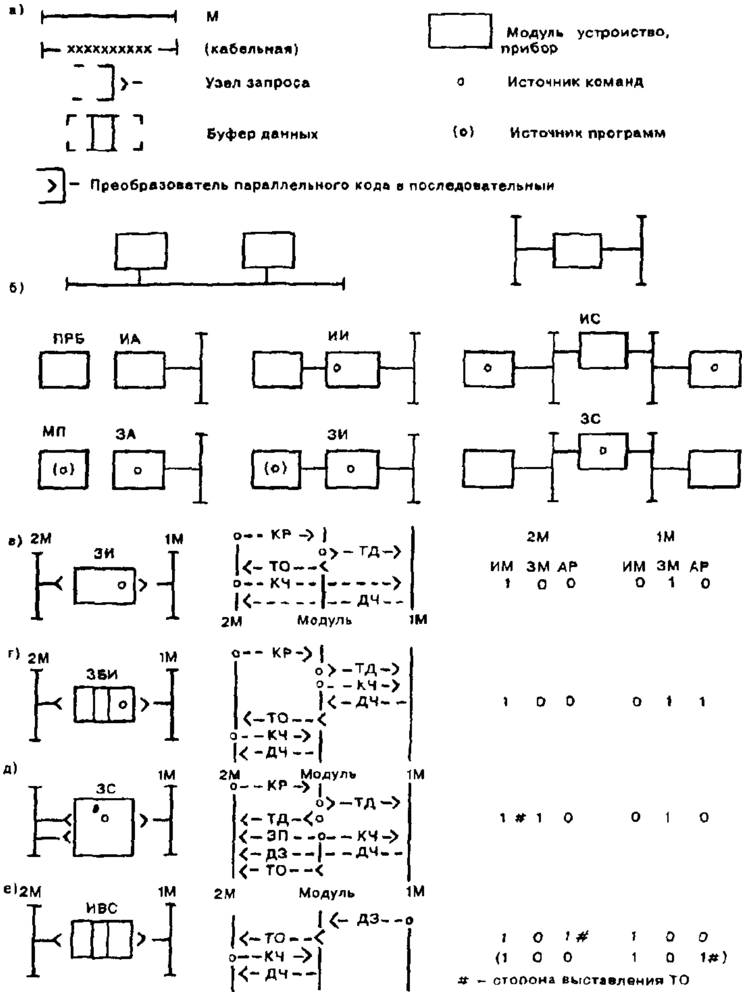
а) основные функциональные элементы МСИ б) основные типы узличков и исполнители типичные работы в) ЗИ г) ЗИ с буфером данных д) ЗС е) ИС с буфером данных
