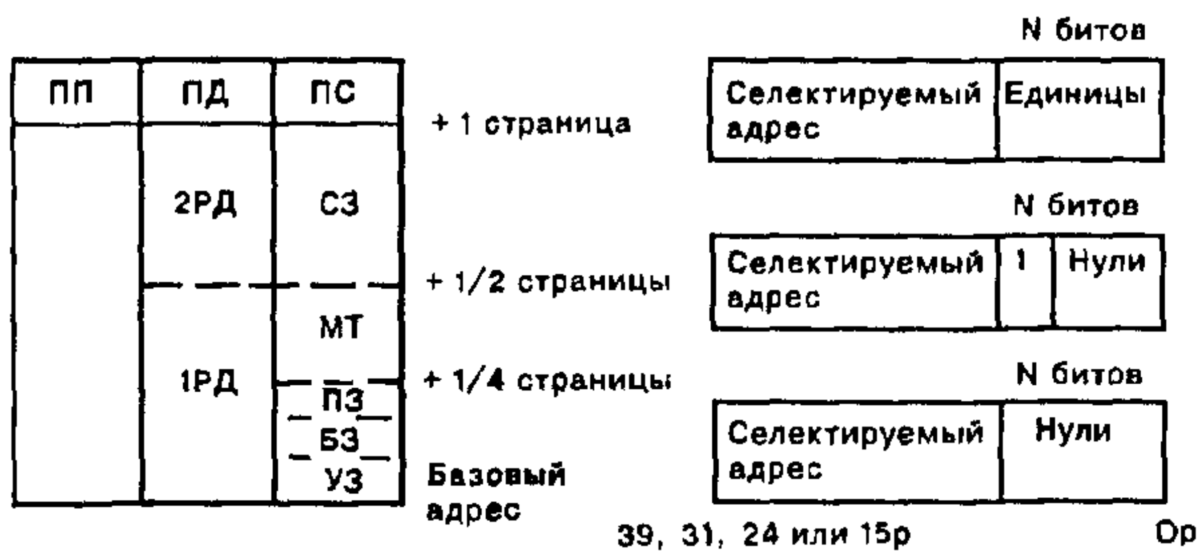
Рисунок Б.10 — Расположение регистров в зоне ВА модуля
