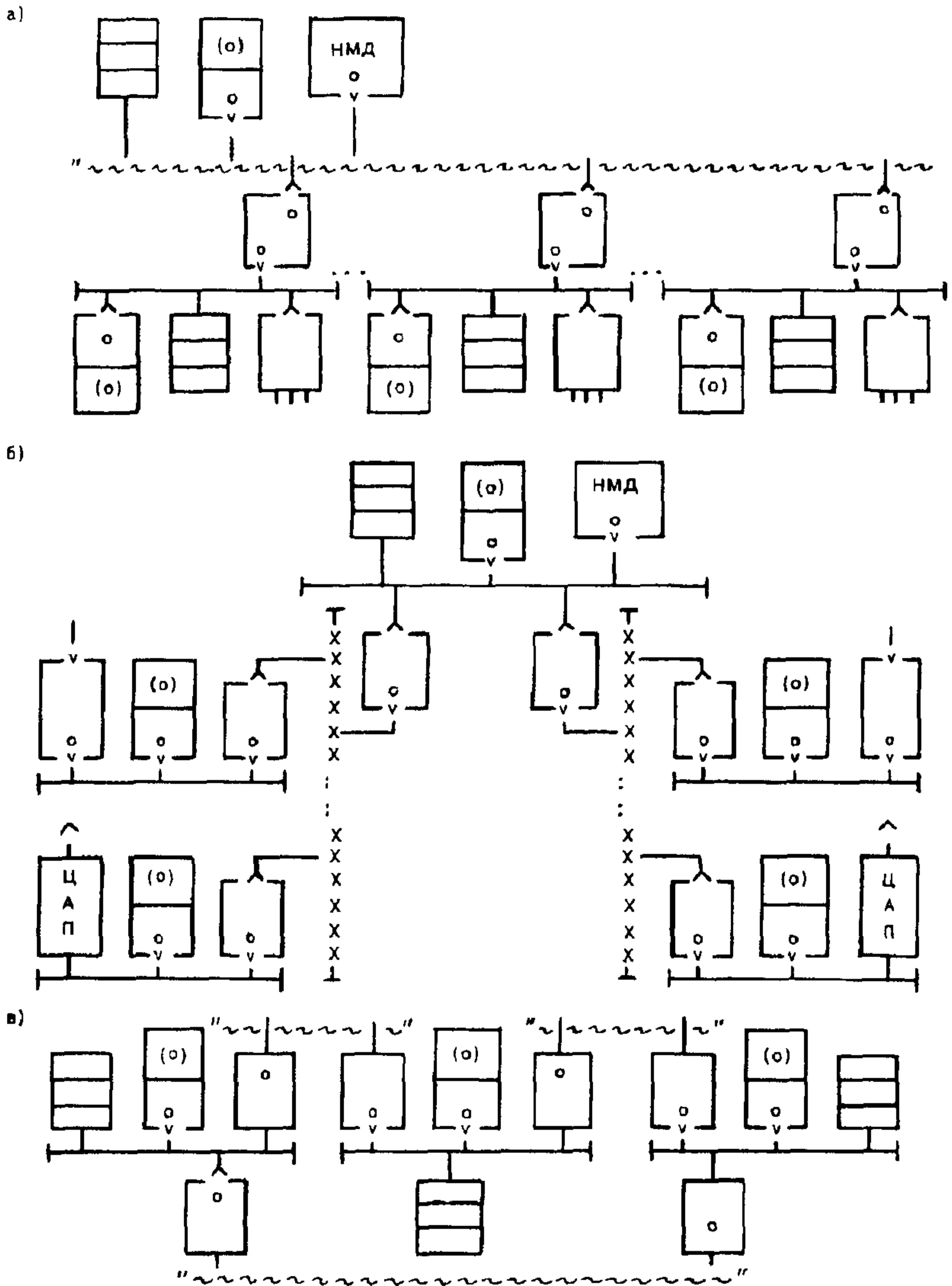
а) двухуровневая линейная структура на основе кабельной межкаркасной магистрали б) трехуровневая древовидная структура в) кольцевая структура
