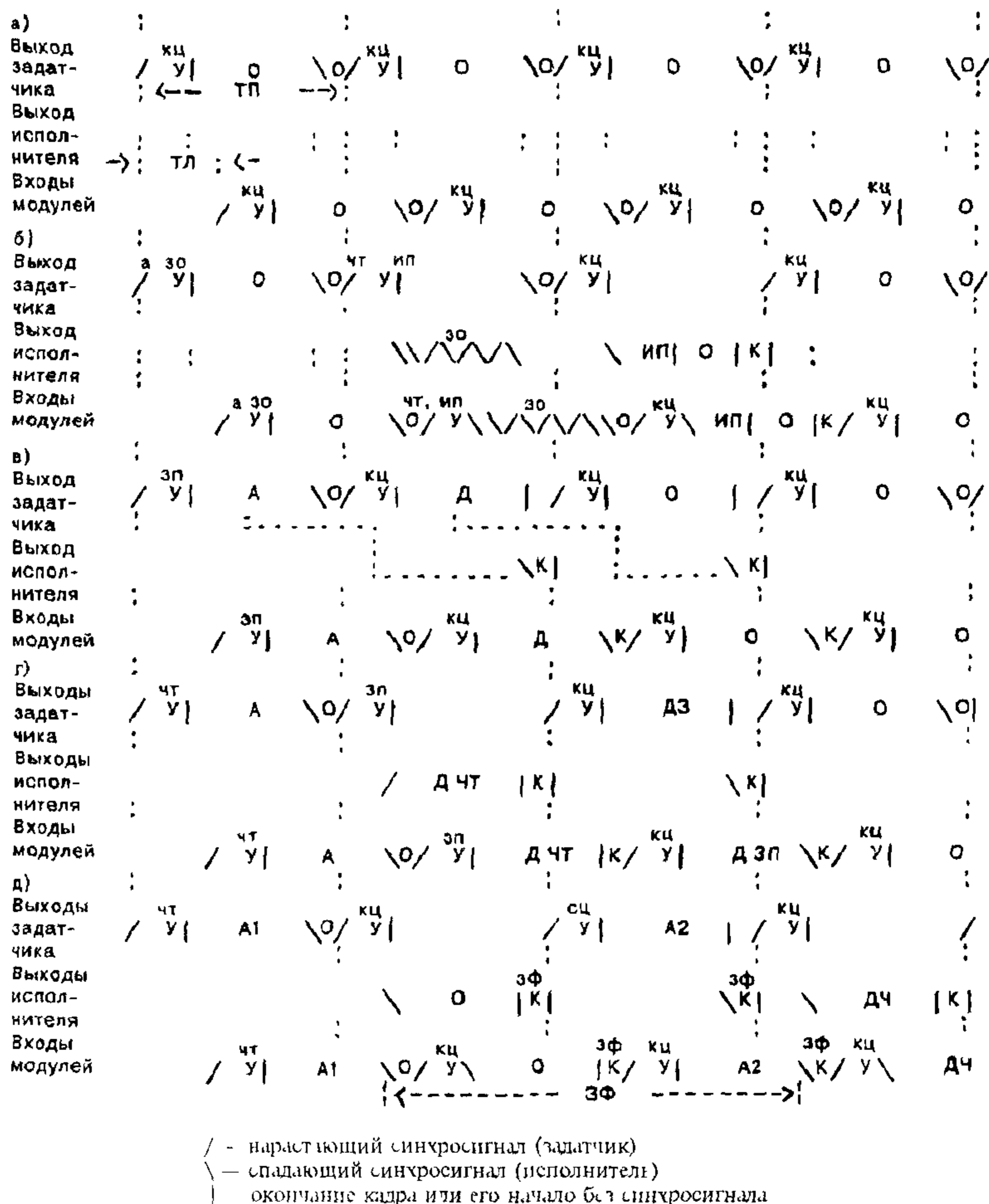
а) свободная магистраль б) цикл арбитража приоритетов зо в) единичный цикл записи данных г) единичный цикл чтения данных д) цикл чтения данных с задержкой фазы передачи
