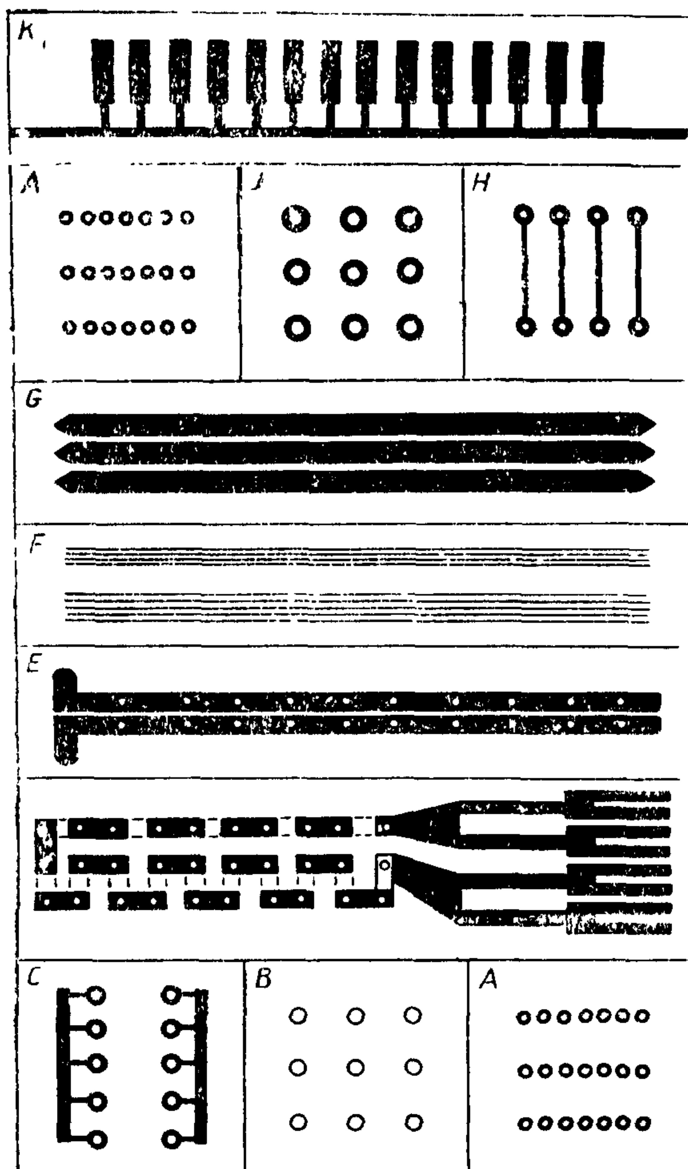
Рисунок 1б — Составной рисунок для испытаний (оборотная сторона)
