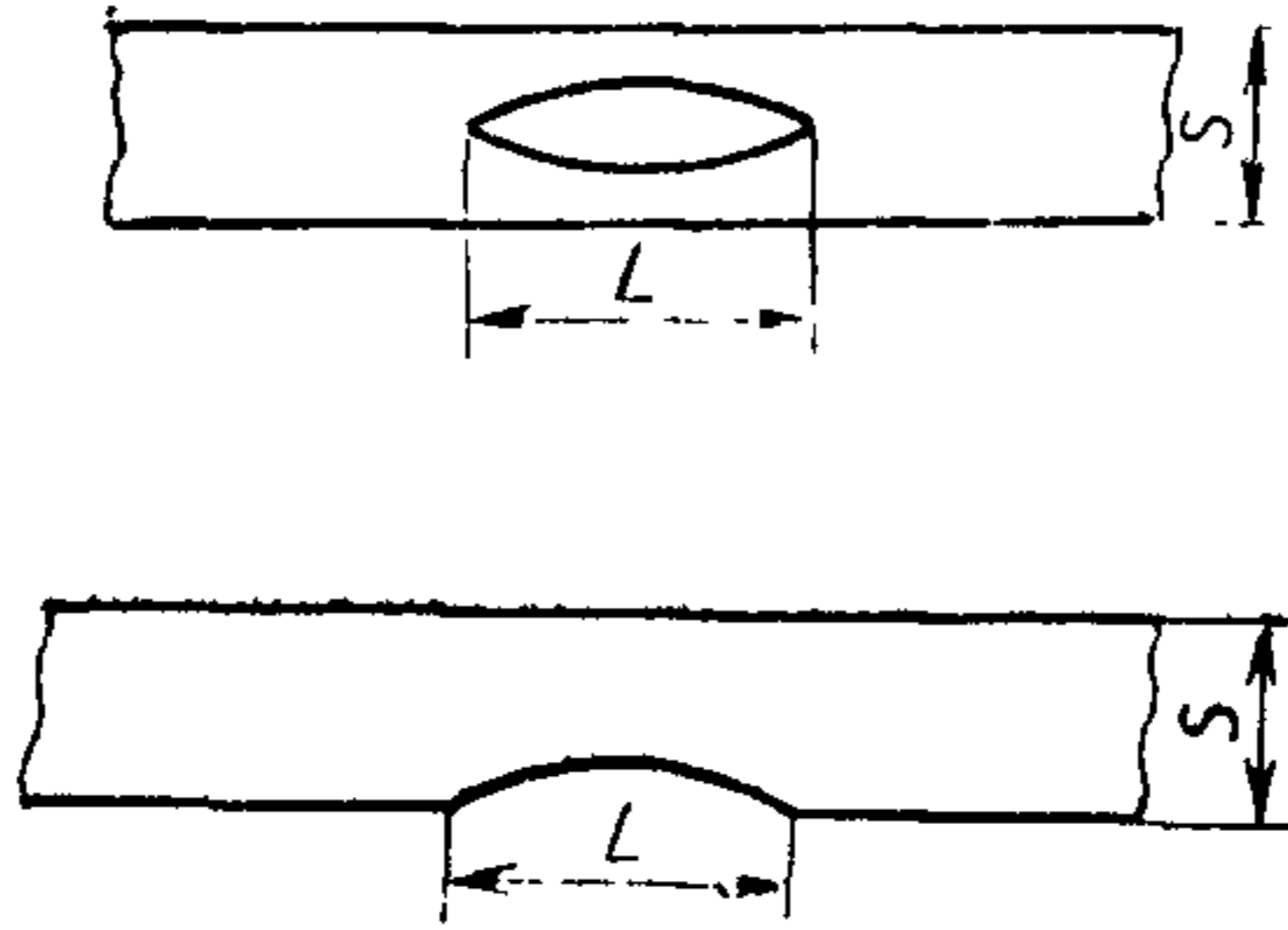
Рисунок 2 — Длина дефекта
