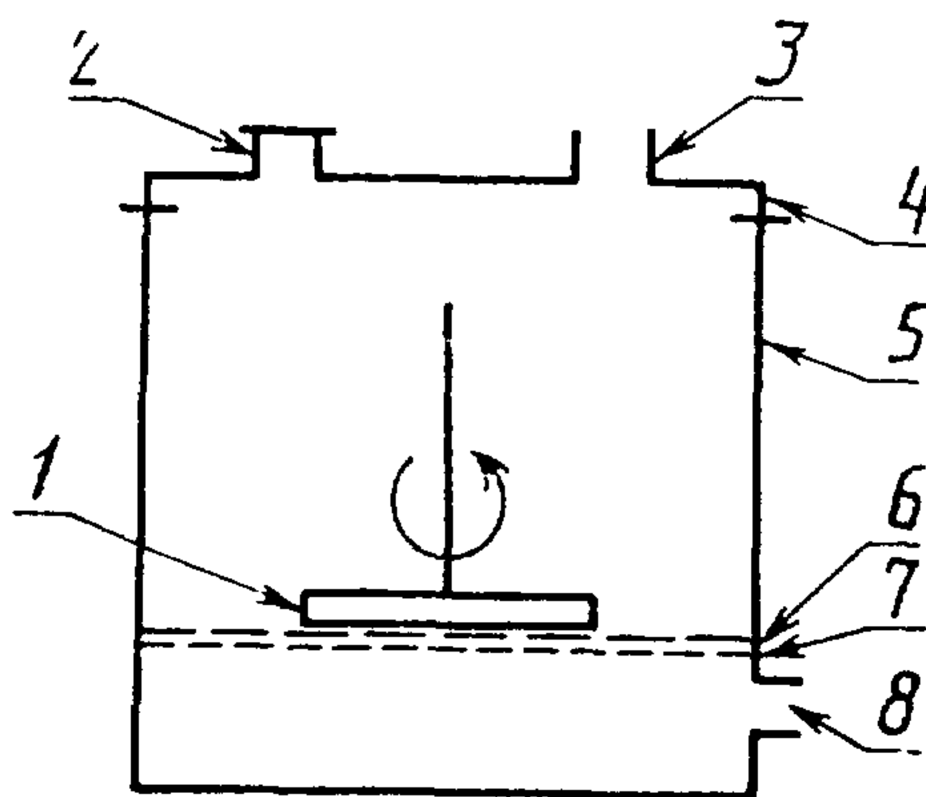
Условное изображение ячейки для определения производительности мембран
