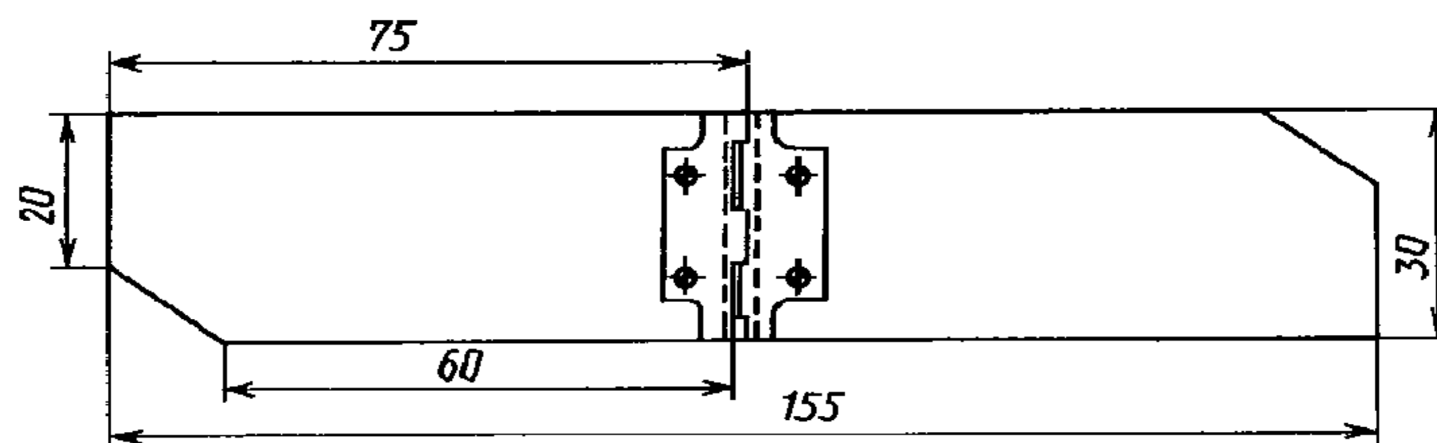
Рисунок 2 — Давящая пластинка
