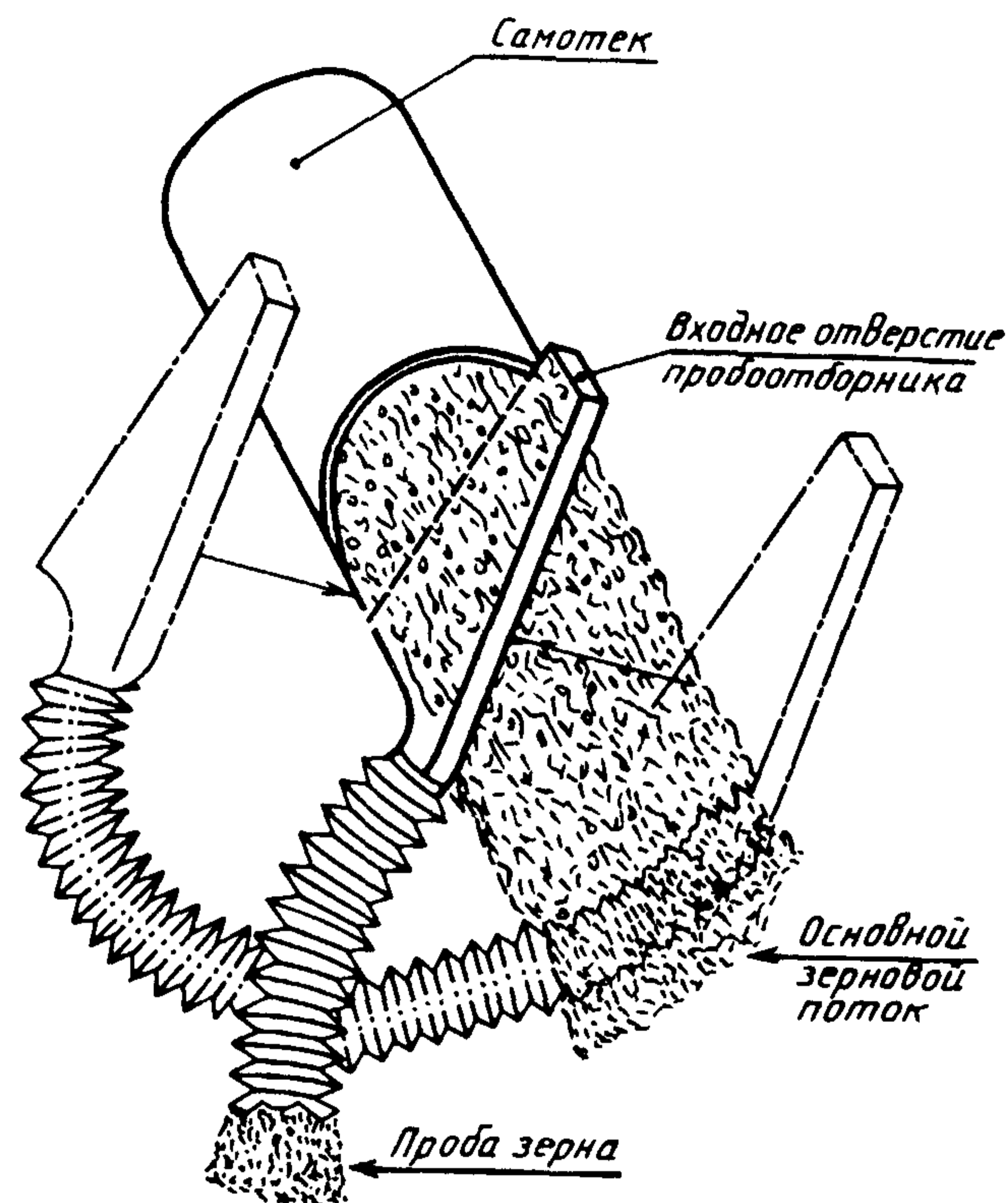
Рисунок 1 — Автоматический пробоотборник отклоняющегося типа для периодического и непрерывного отбора проб
