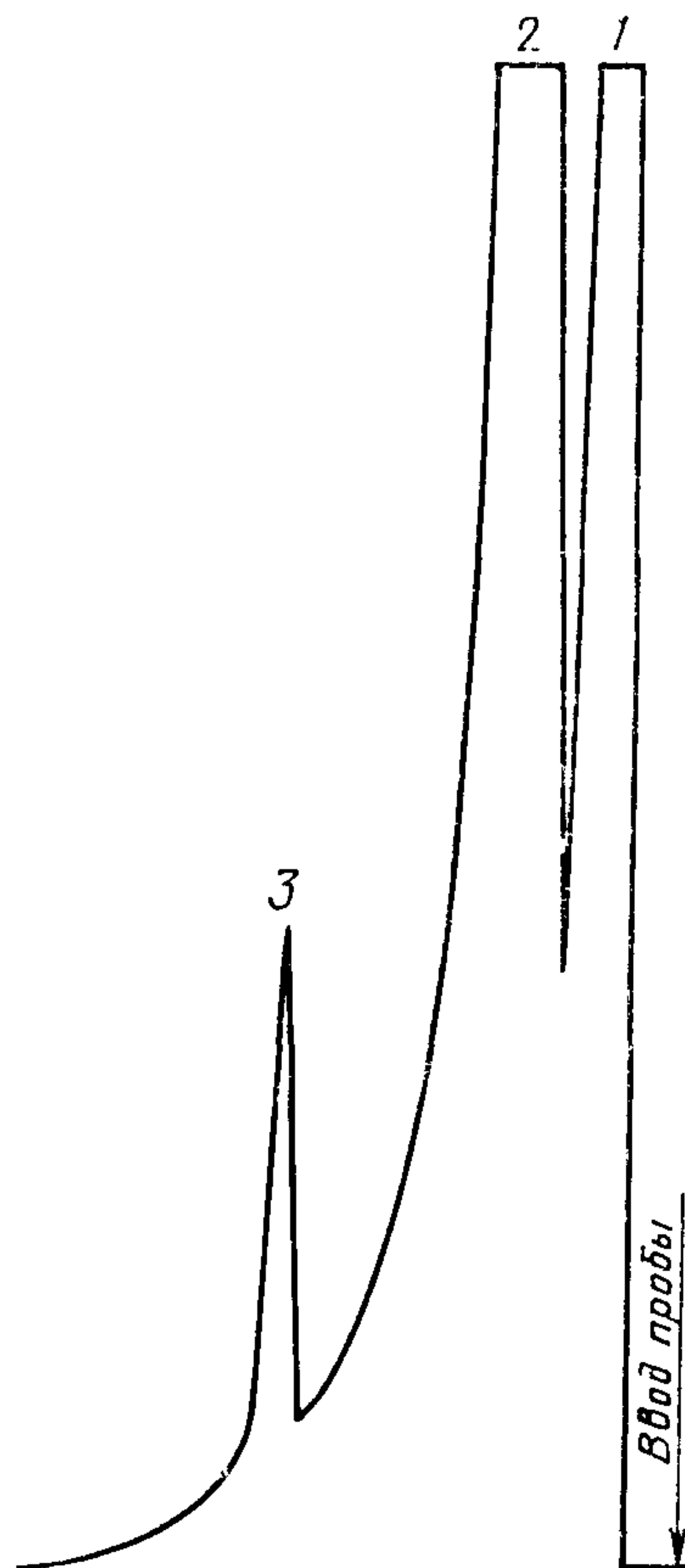
1 — ацетон; 2 — 4-хлорнитробензол; 3 — 2,4-динитрохлорбензол
