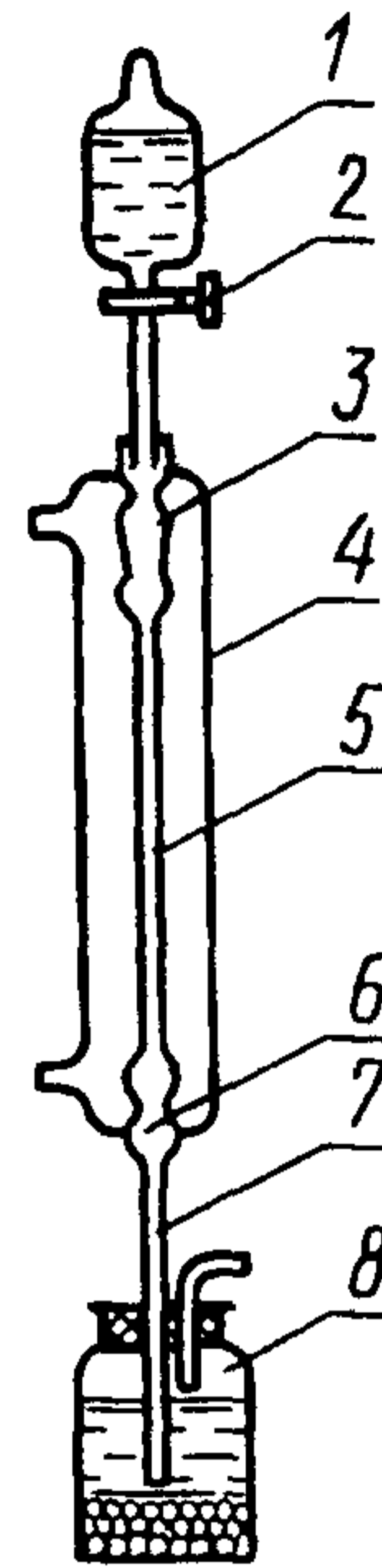
Капиллярный вискозиметр
