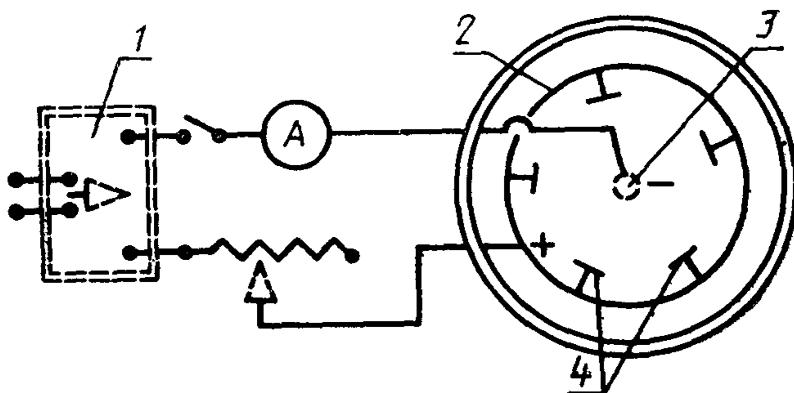
Схема установки катодной очистки пластин
