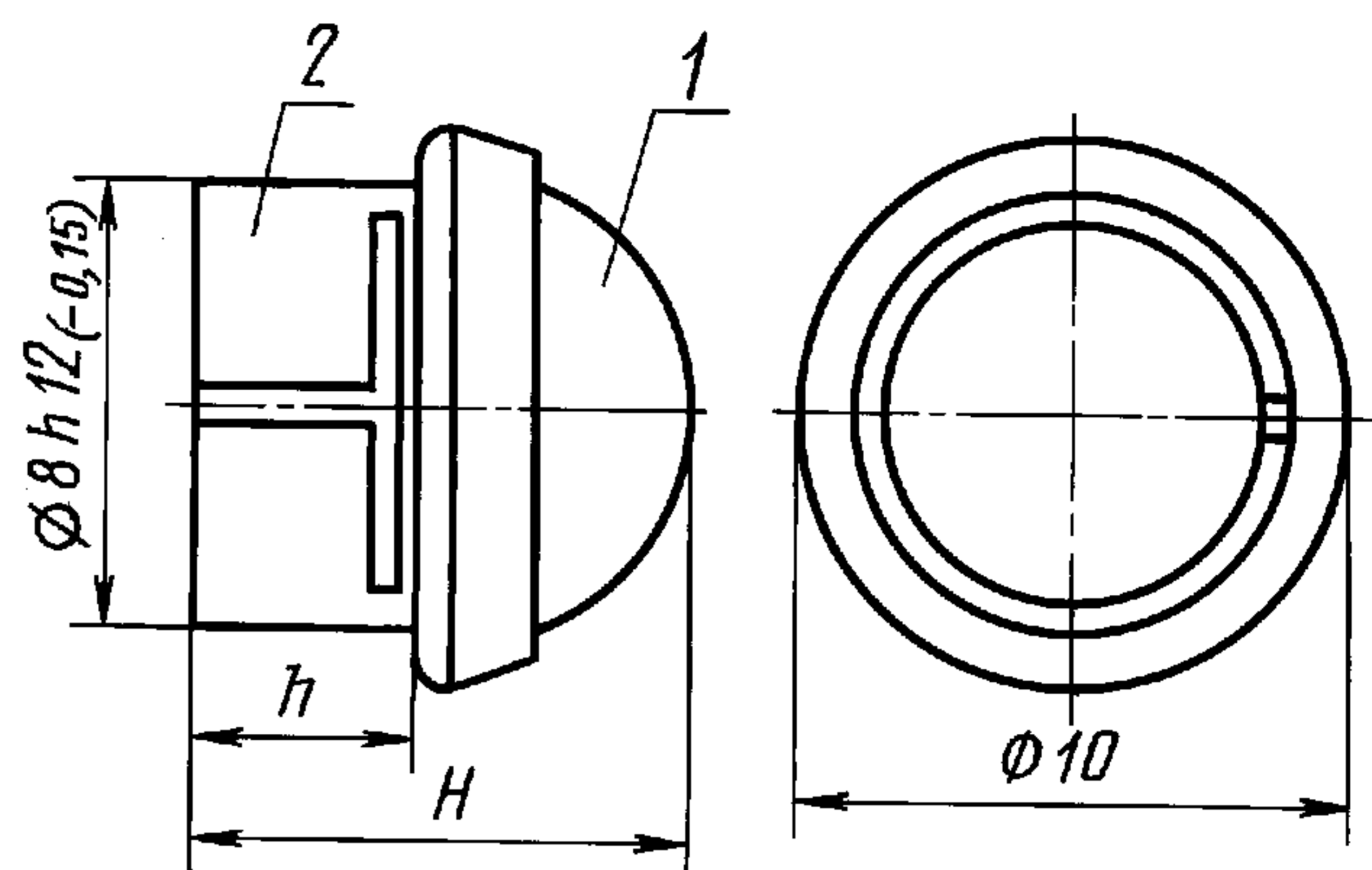
Линза типа Л2
