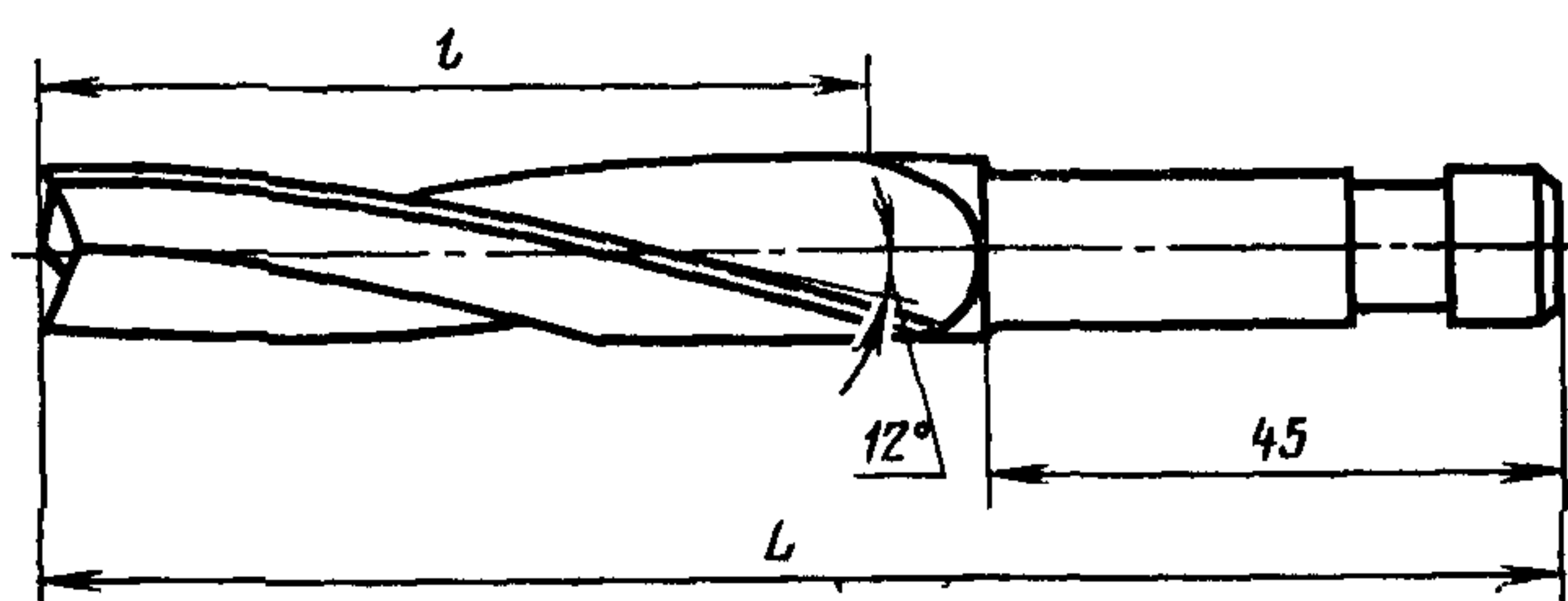
Вариант изготовления фрез типа 2 с винтовой канавкой
