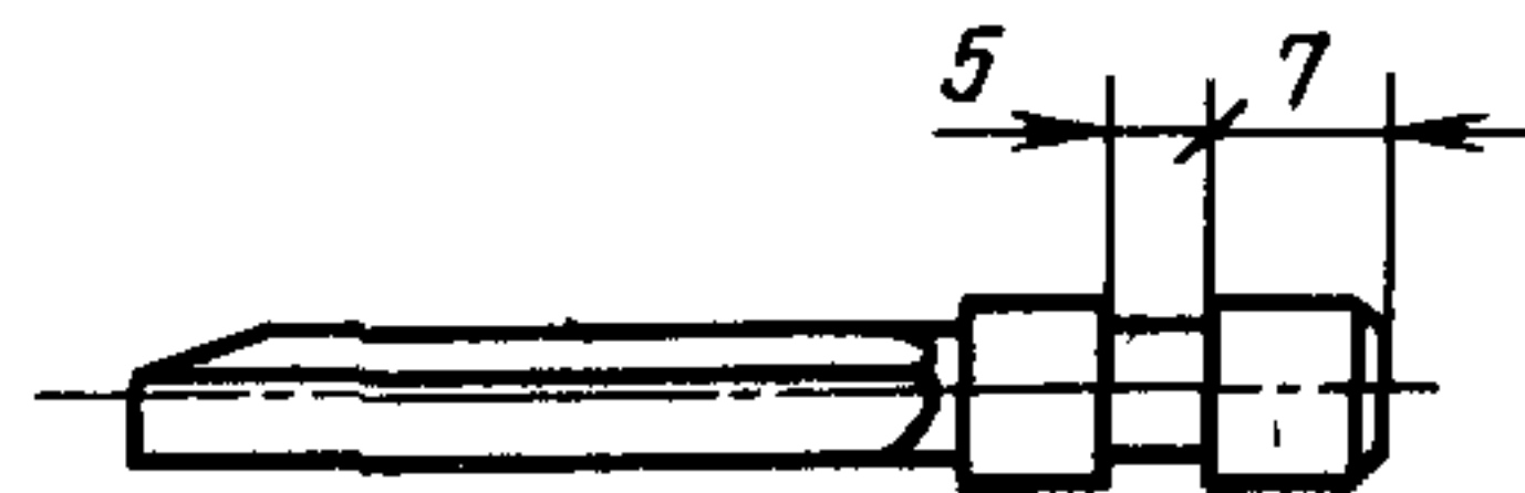
Допустимый вариант исполнения хвостовика для фрез D = 4 мм
