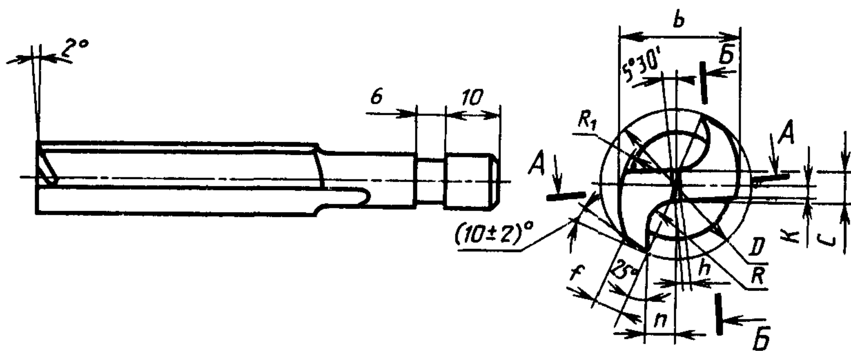
Фреза типа 2 с прямой канавкой
