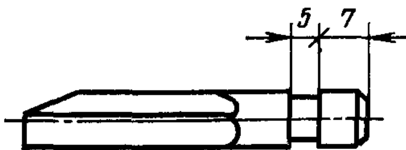
Исполнение хвостовика фрез размером D = 4 мм
