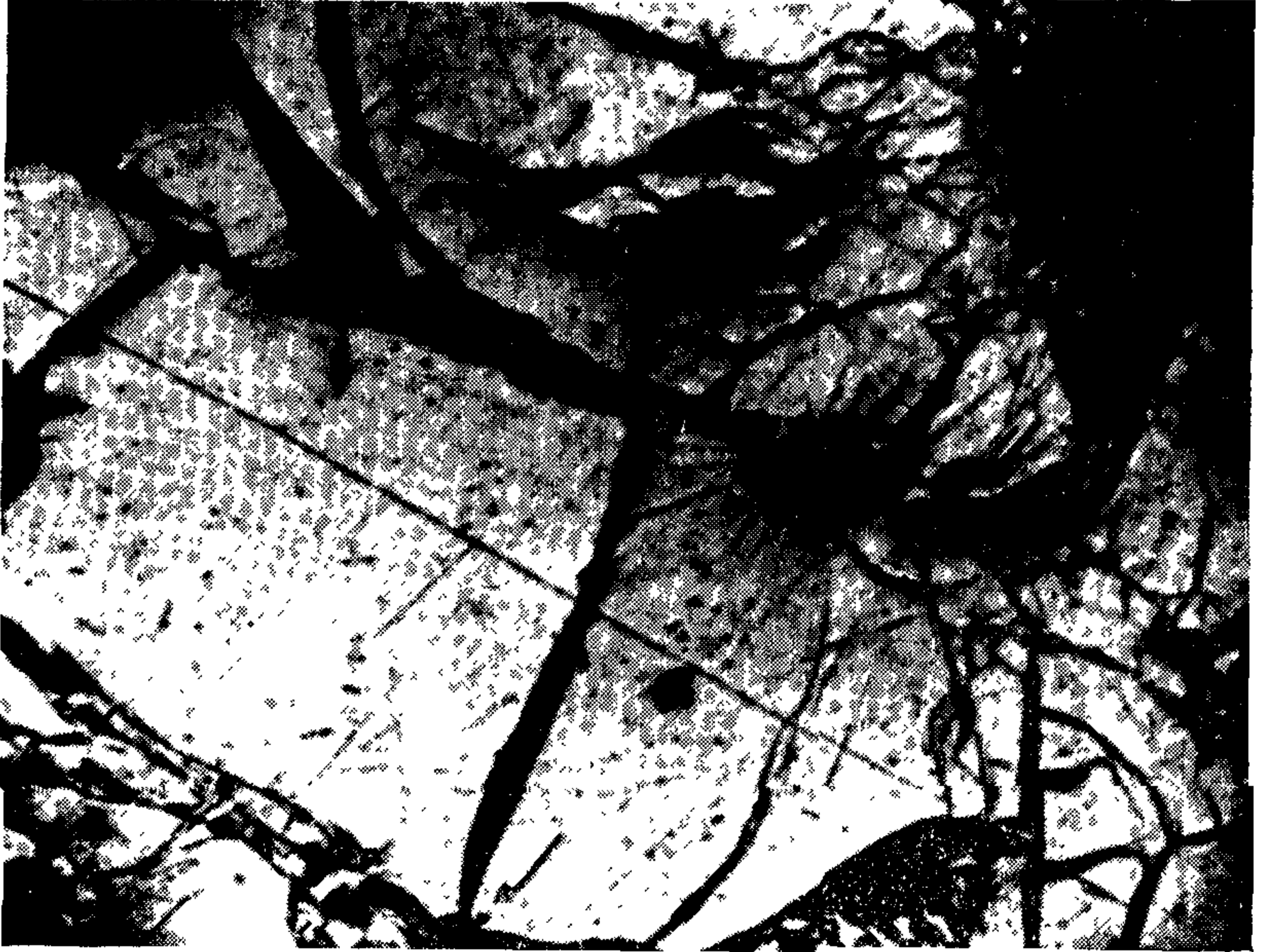
Высокая степень выветрелости угля. Появление дезинтеграции частиц угля и пустот выщелачивания
