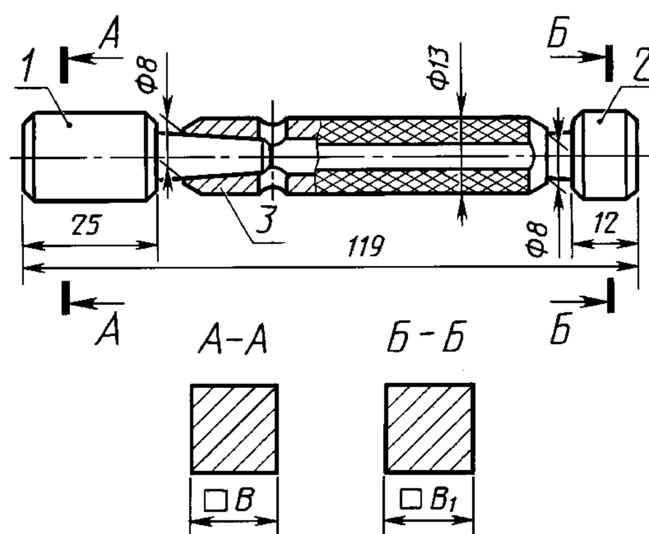
1 — проходная вставка; 2 — непроходная вставка; 3 — ручка по ГОСТ 14748
