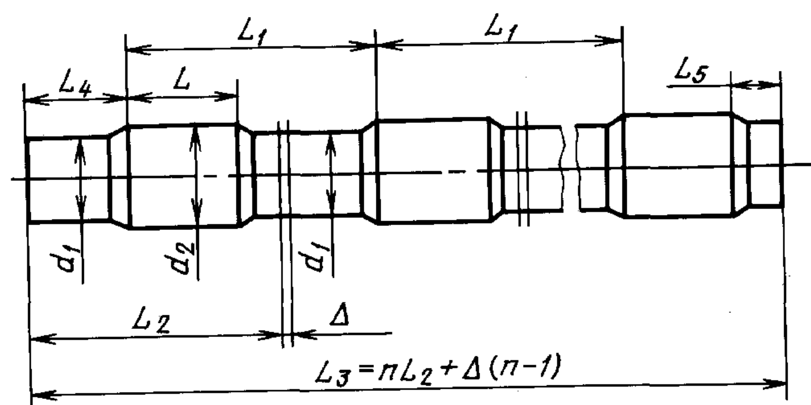
Размеры, мм
