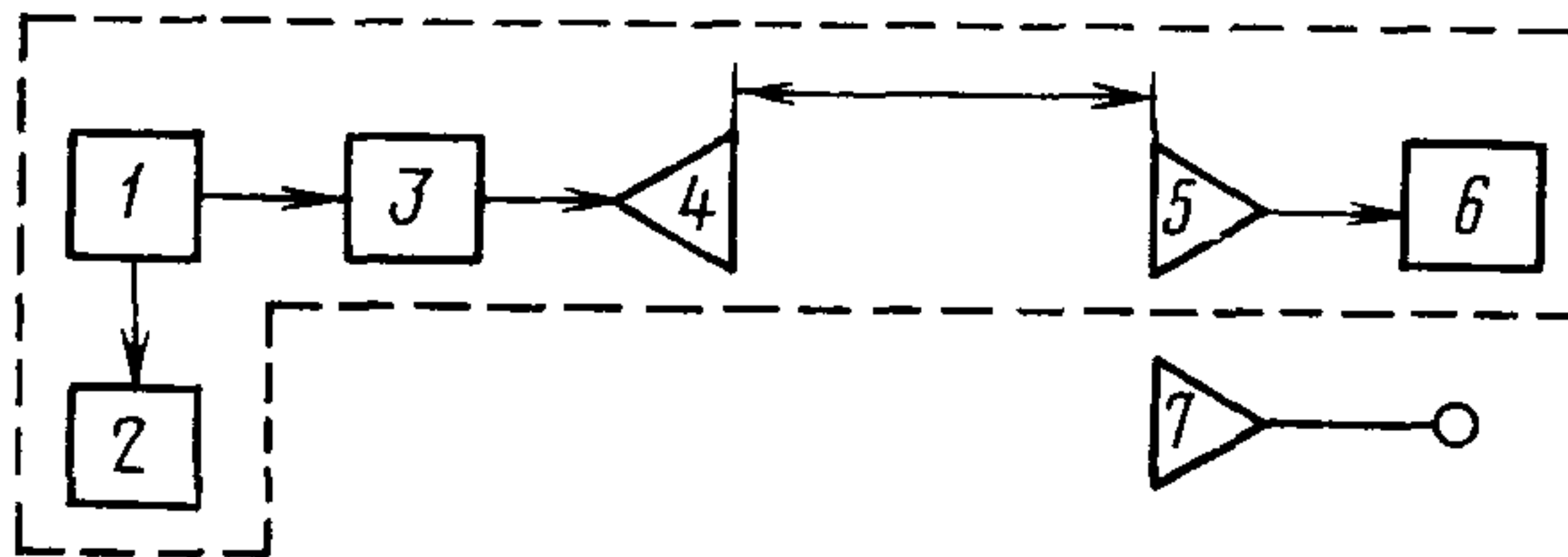
1—генератор сигналов; 2—частотомер; 3—измерительный аттенюатор; 4—вспомогательная антенна; 5—образцовая антенна; 6—измерительный приемник; 7—поверяемая антенна
