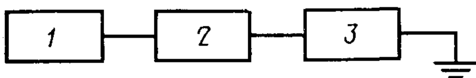
1—генератор; 2—измерительная секция образцового амперметра; 3—поверяемый амперметр
