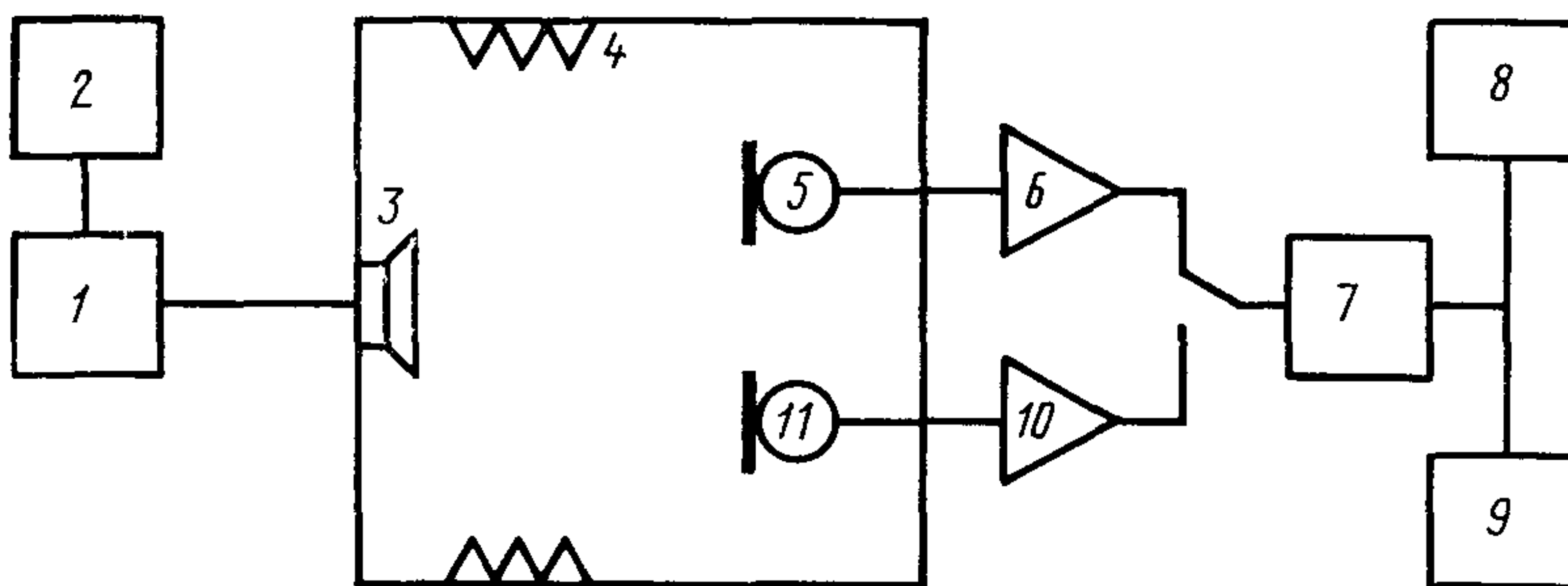
1—генератор, 2—частотомер; 3—громкоговоритель, 4—заклушенная камера, 5 и 11—образцовый и проверяемый микрофоны, 6 и 10—микрофонные усилители, 7—магазин затухания, 8—электронный вольтметр, 9—осциллограф
