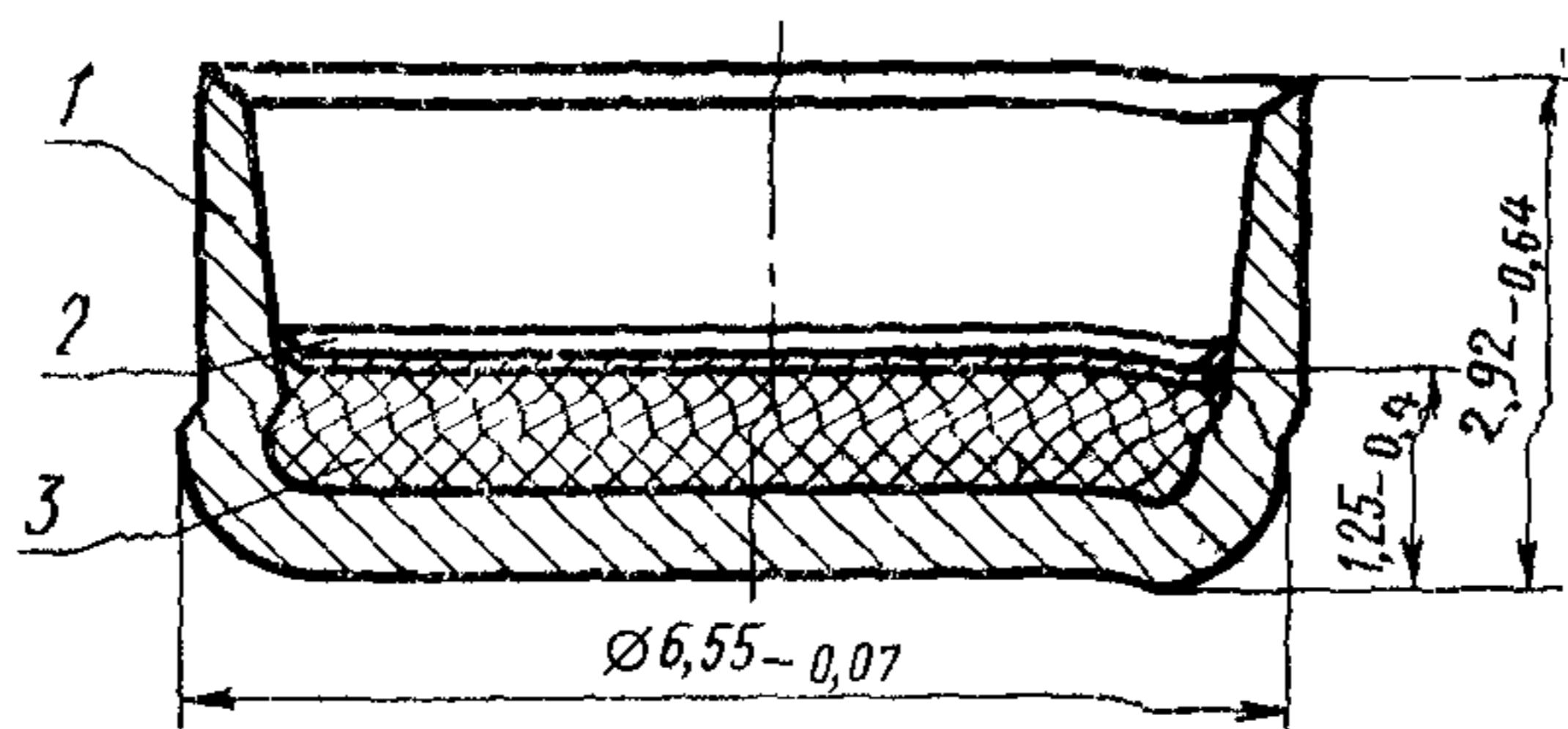
1 — колпачок, 2 — кружок, 3 — состав ударный Черт. 1
