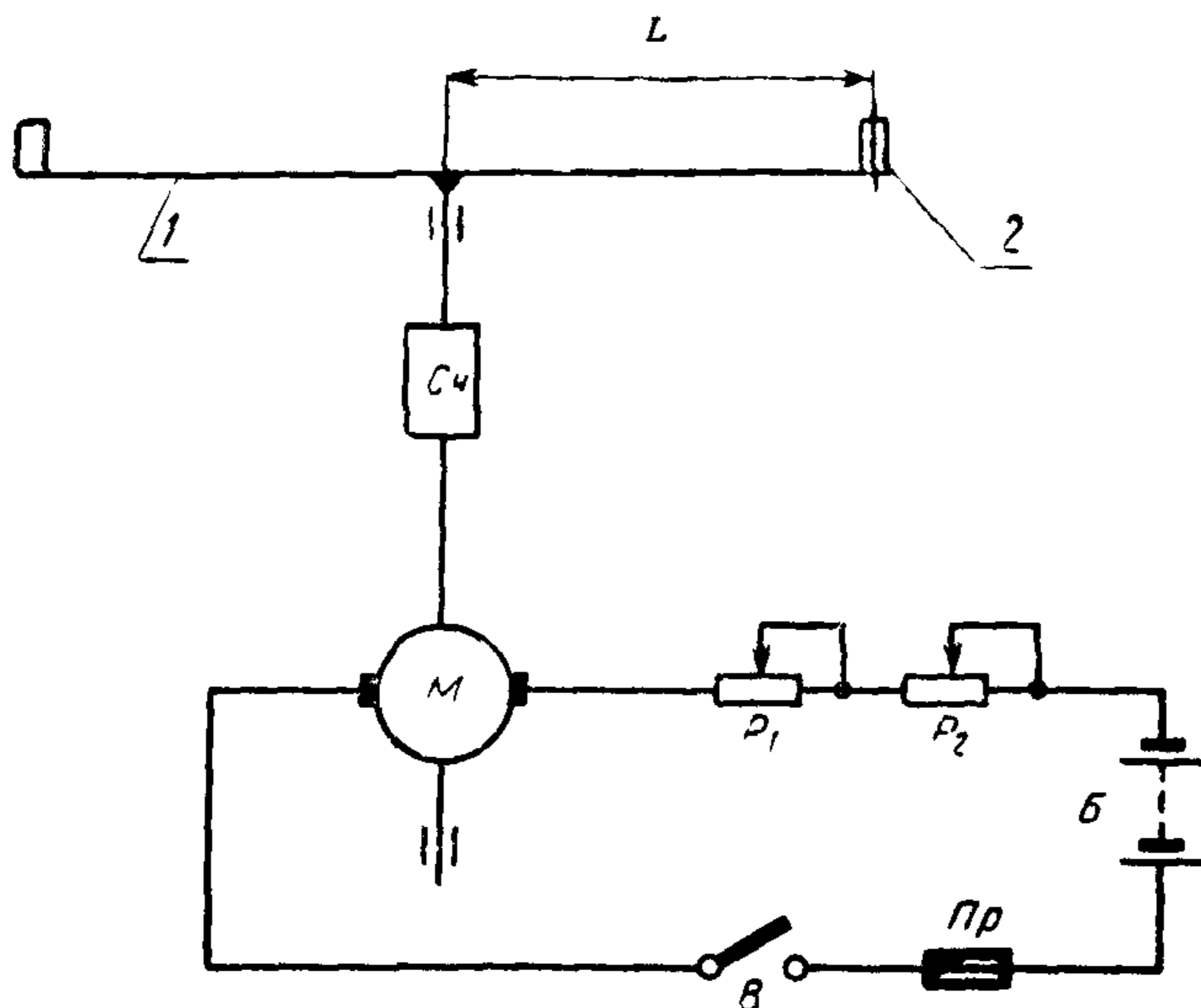
1—крестовина 2—стойка для крепления проверяемых анемометров, Сч—счетчик числа оборотов крестовины М—двигатель Р 1 Р 2 —реостаты Б—аккумуляторная батарея В—выключатель Пр предохранитель
