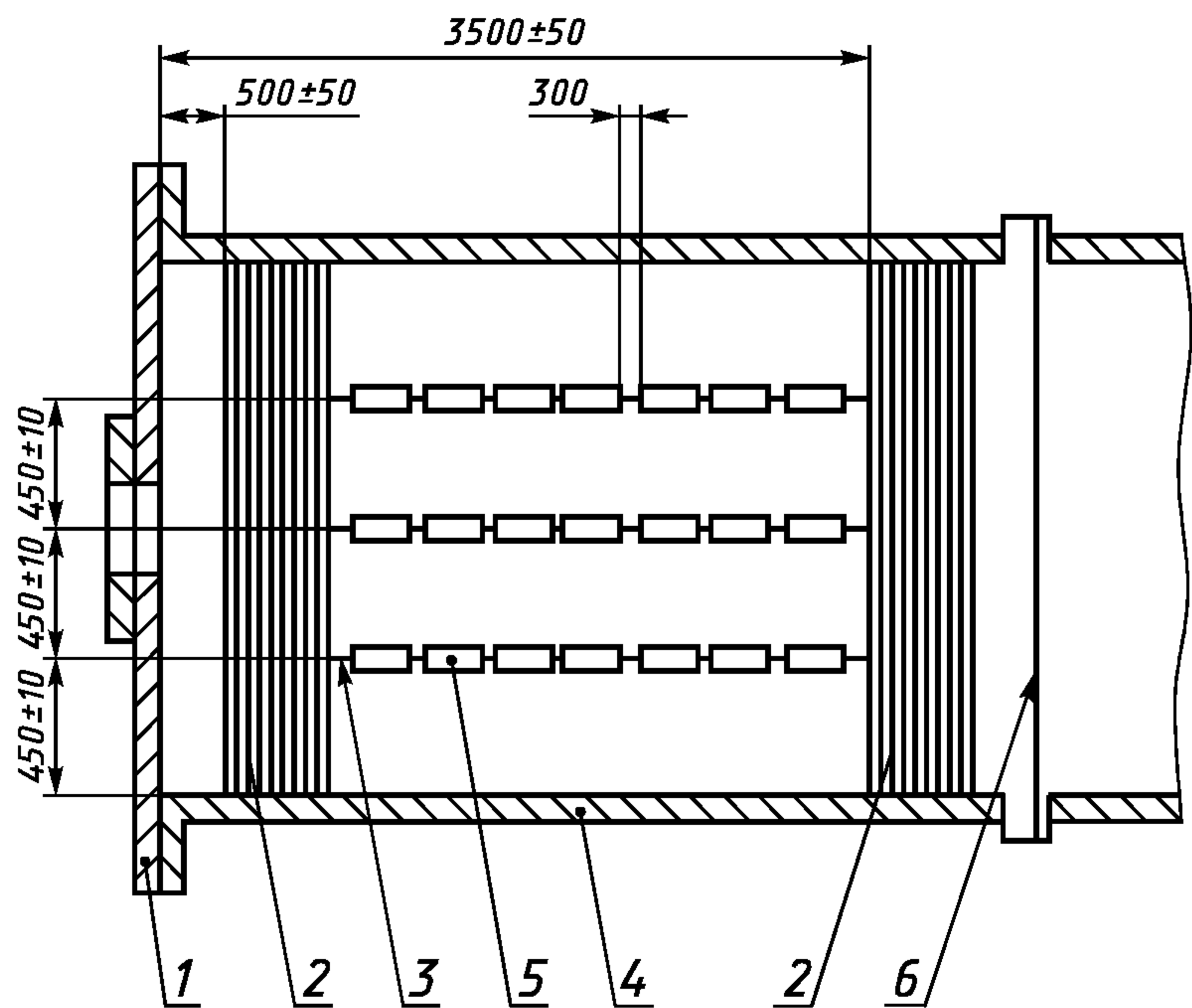
1 — днище трубы штрека; 2 — деревянная рудничная стойка; 3 — капроновая леска или провод; 4 — стенка трубы штрека; 5 — испытуемый заряд ВВ; 6 — диафрагма или штормый затвор
