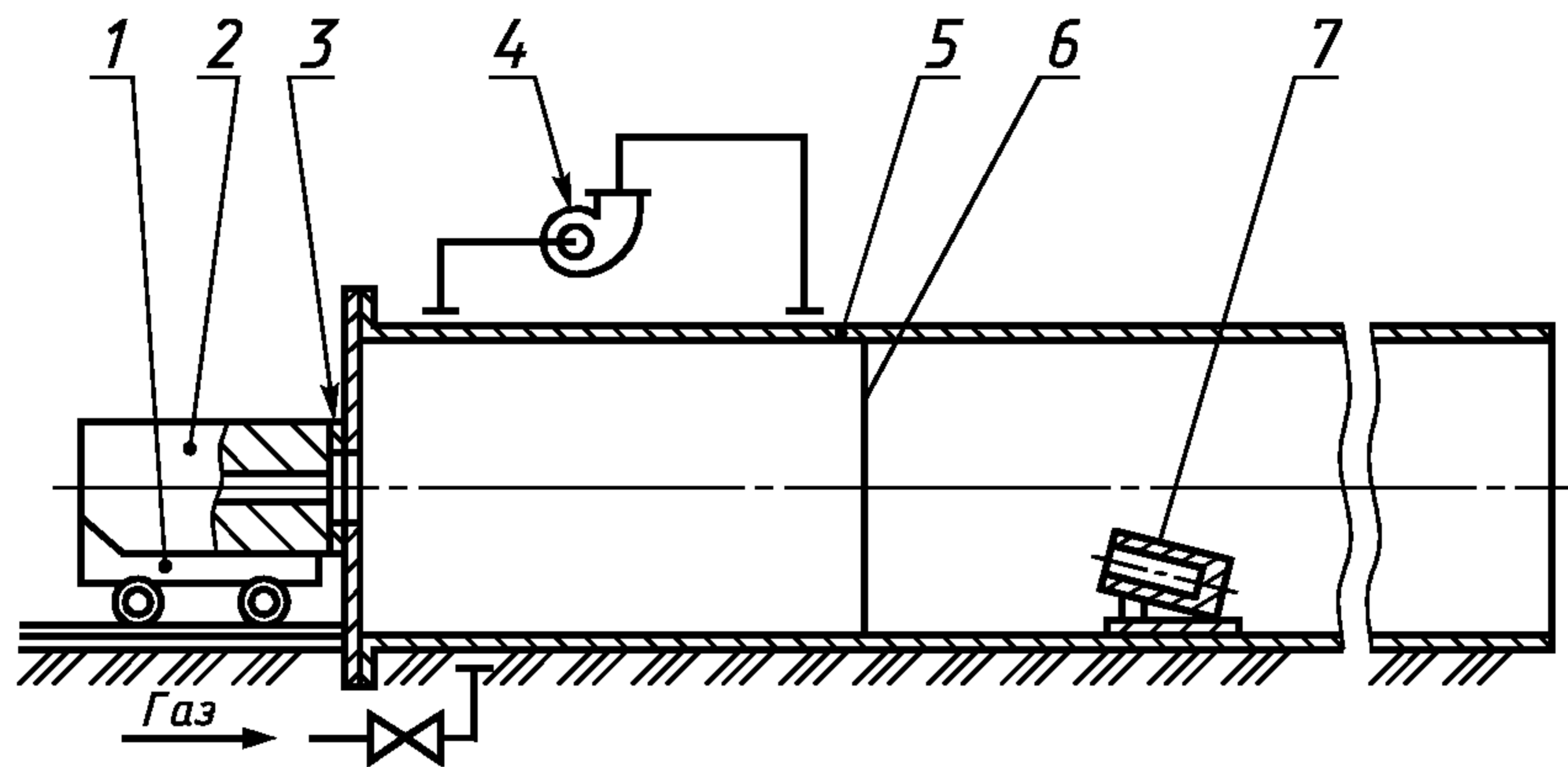
1 — тележка; 2 — каналная мортира; 3 — люк штрека; 4 — вентилятор для перемешивания метановоздушной смеси; 5 — труба штрека; 6 — диафрагма; 7 — мортира для распыления угольной пыли
