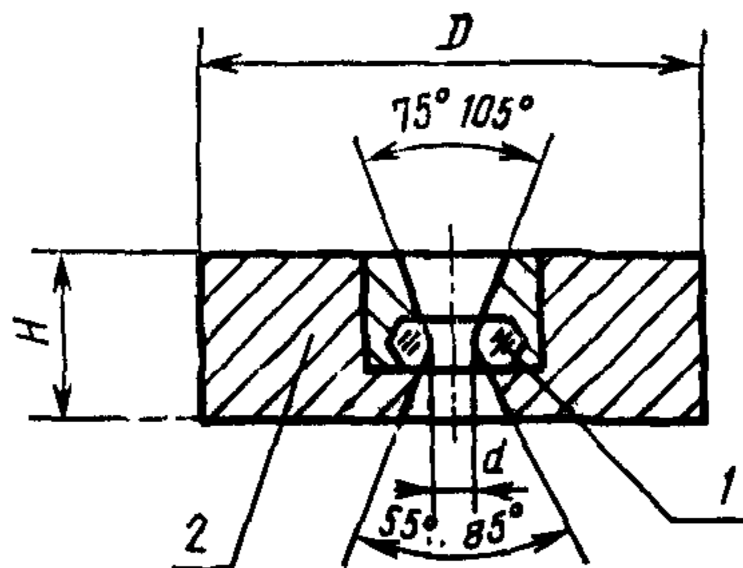
1 — алмаз; 2 — оправка; d — диаметр калибрующего отверстия
