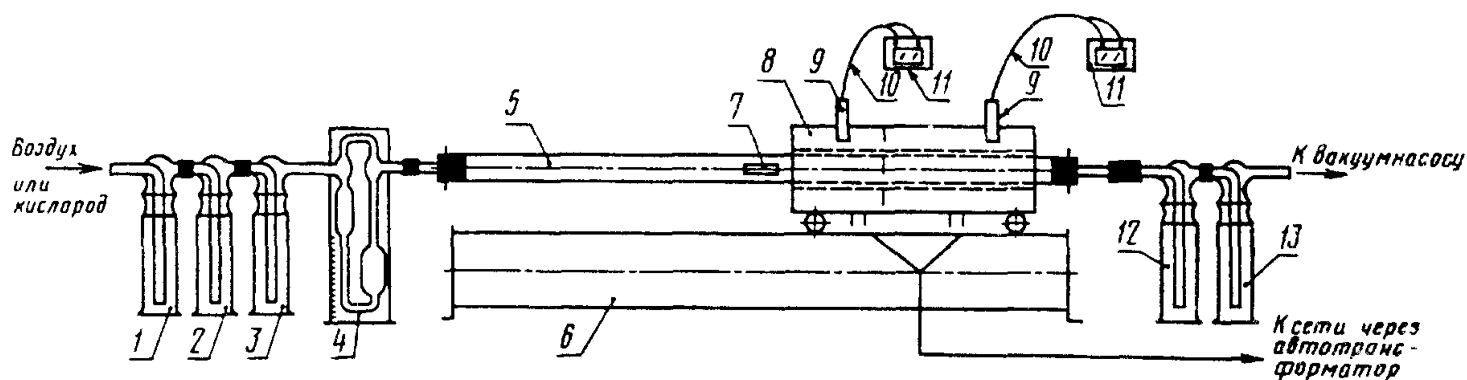
Прибор для определения серы
