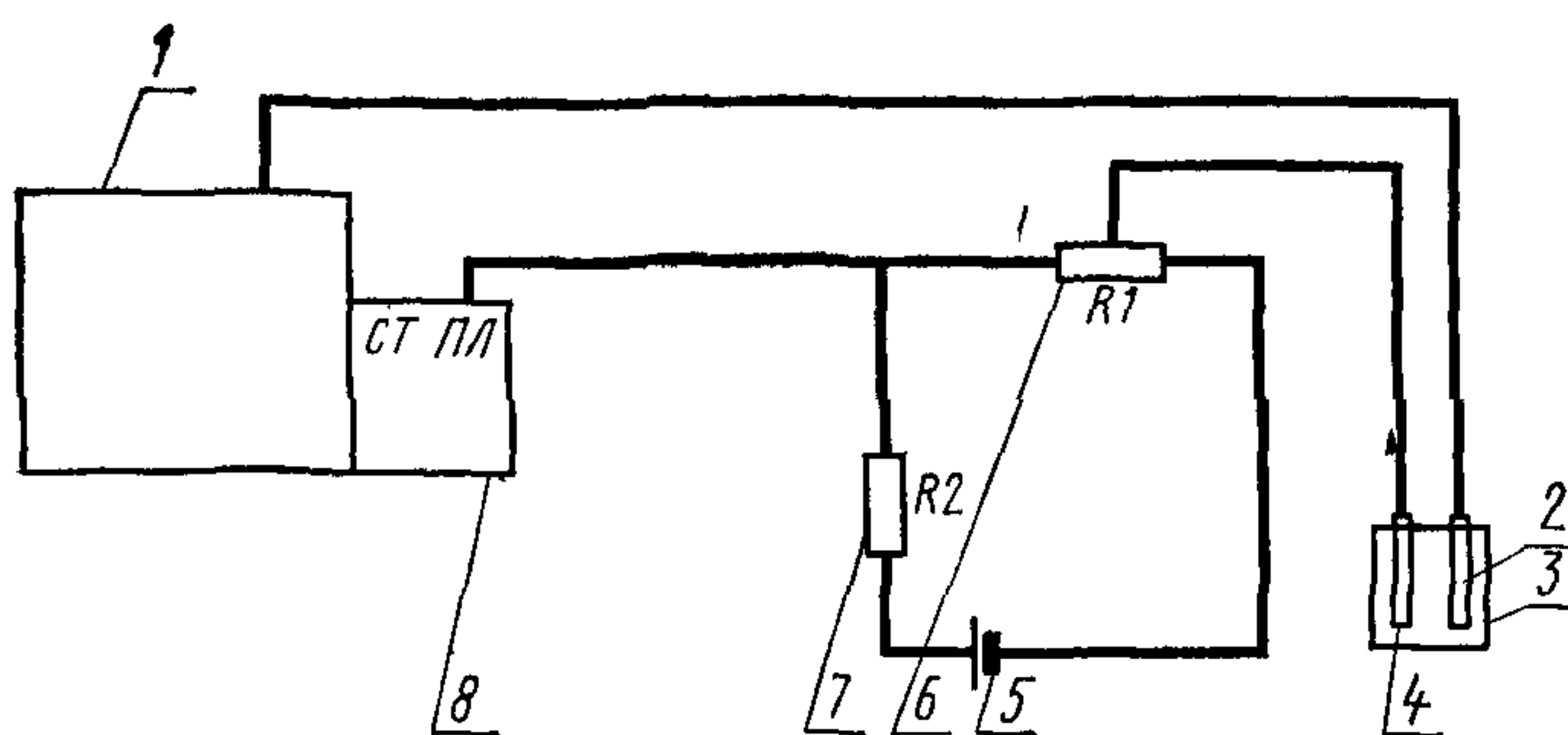
Схема цепи серебряного электрода
