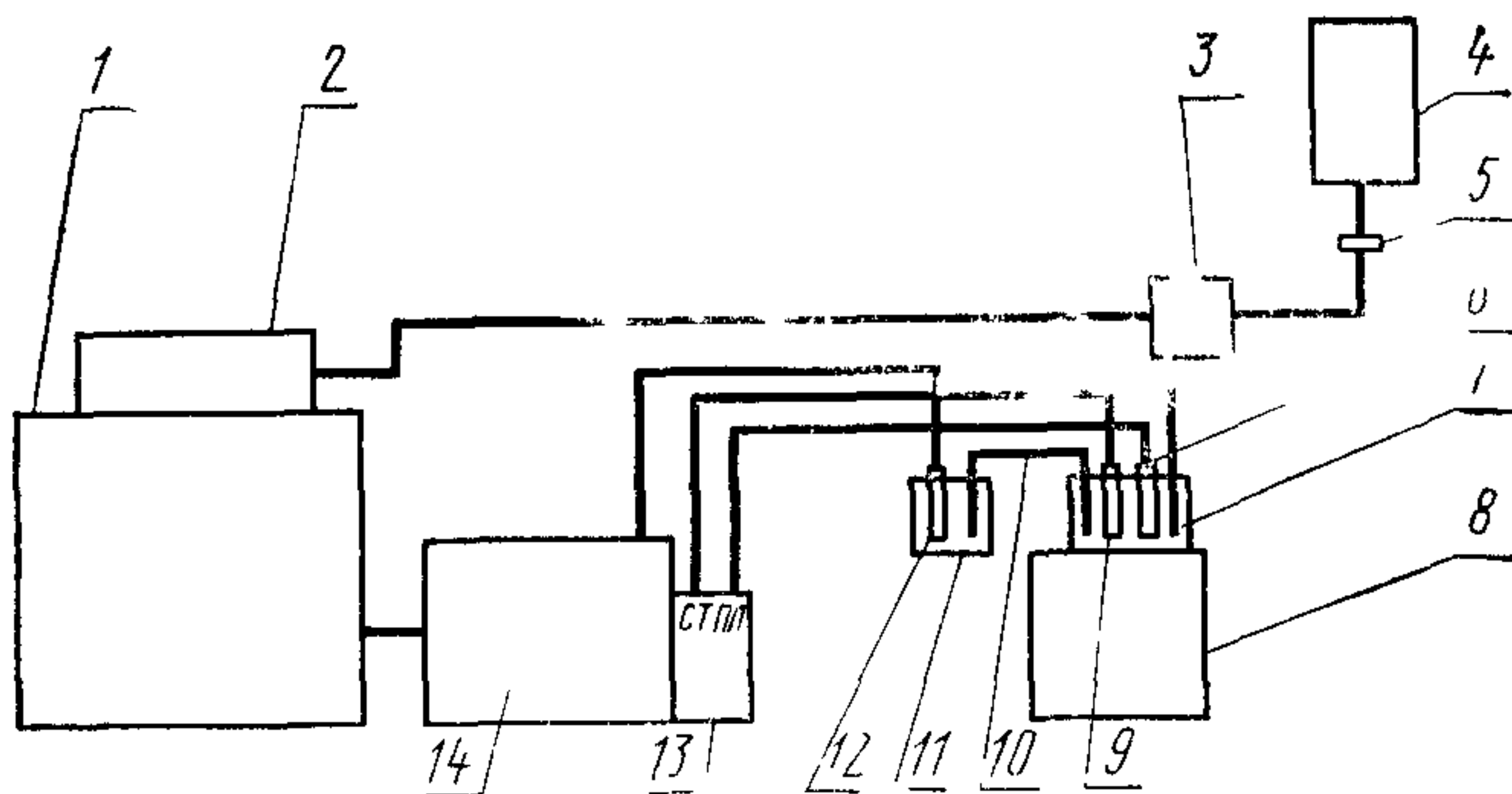
Схема установки автоматического титрования
