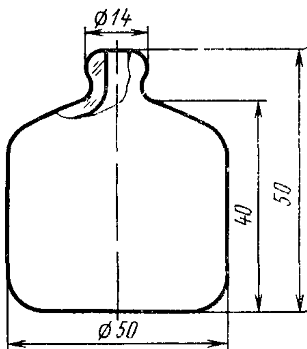
Склянка для омыления в бомбах прибора ЛСАРТ
