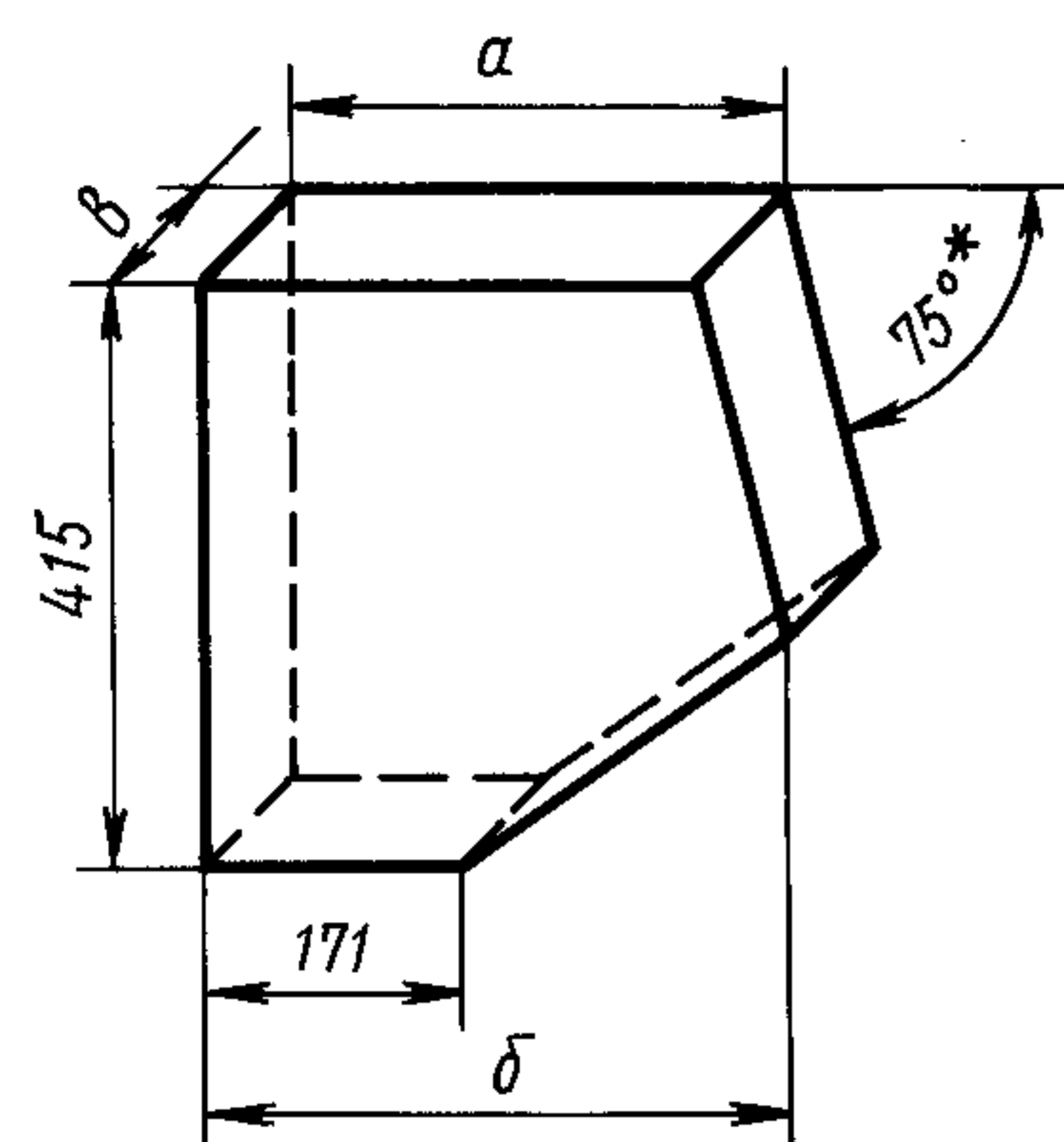
Кирпич поднасадочный пятовый
