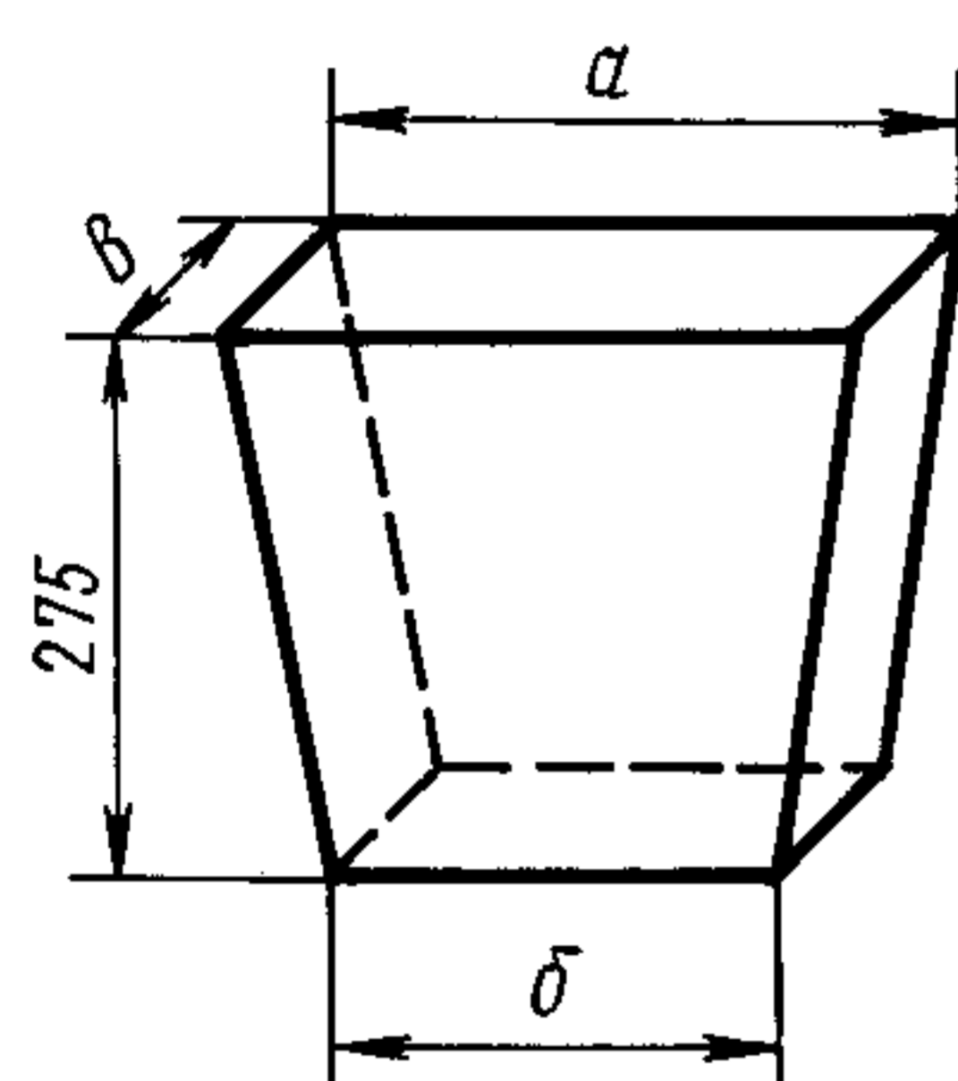
Кирпич поднасадочный распорный
