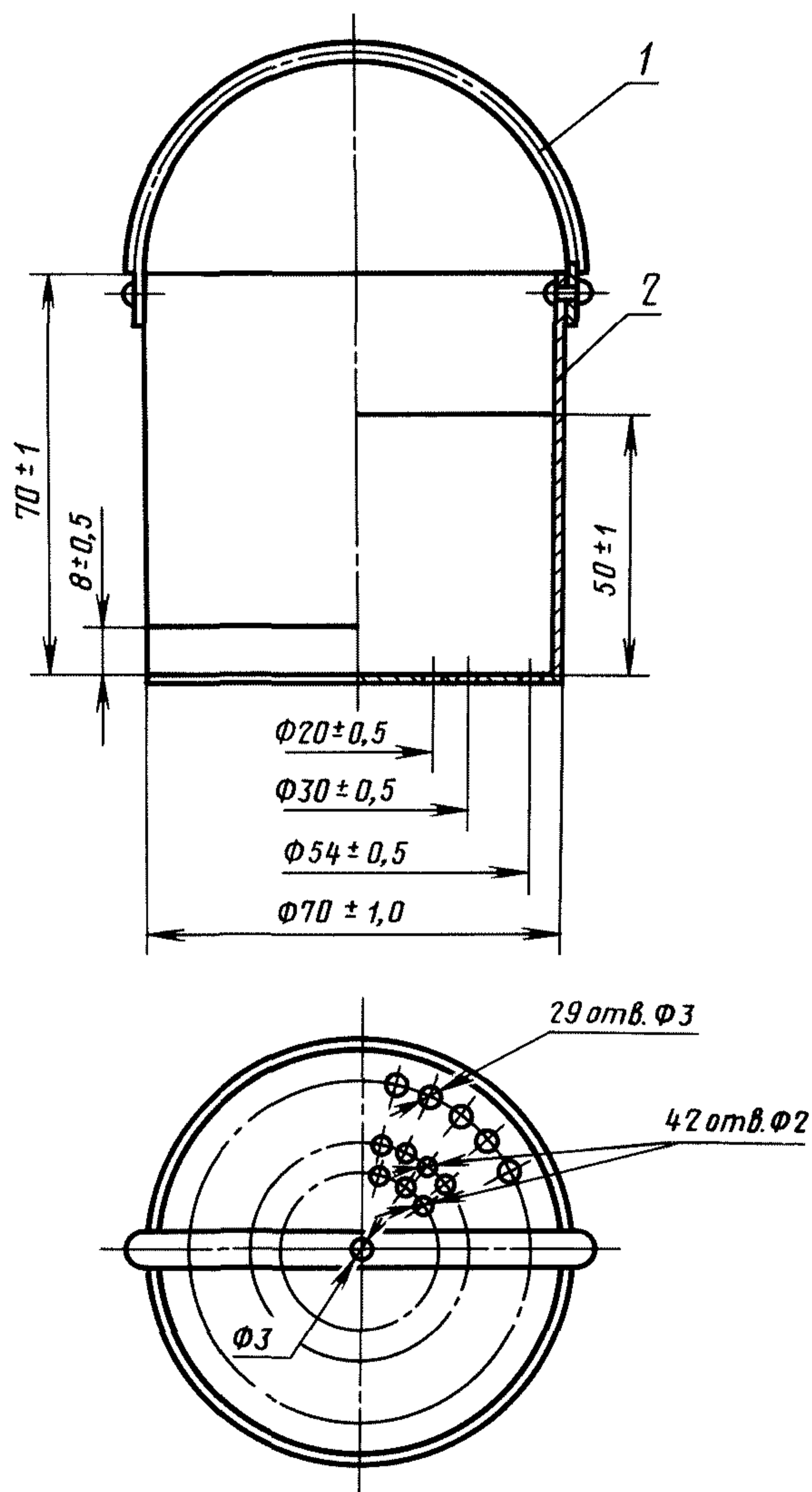
1 — ручка; 2 — корпус
