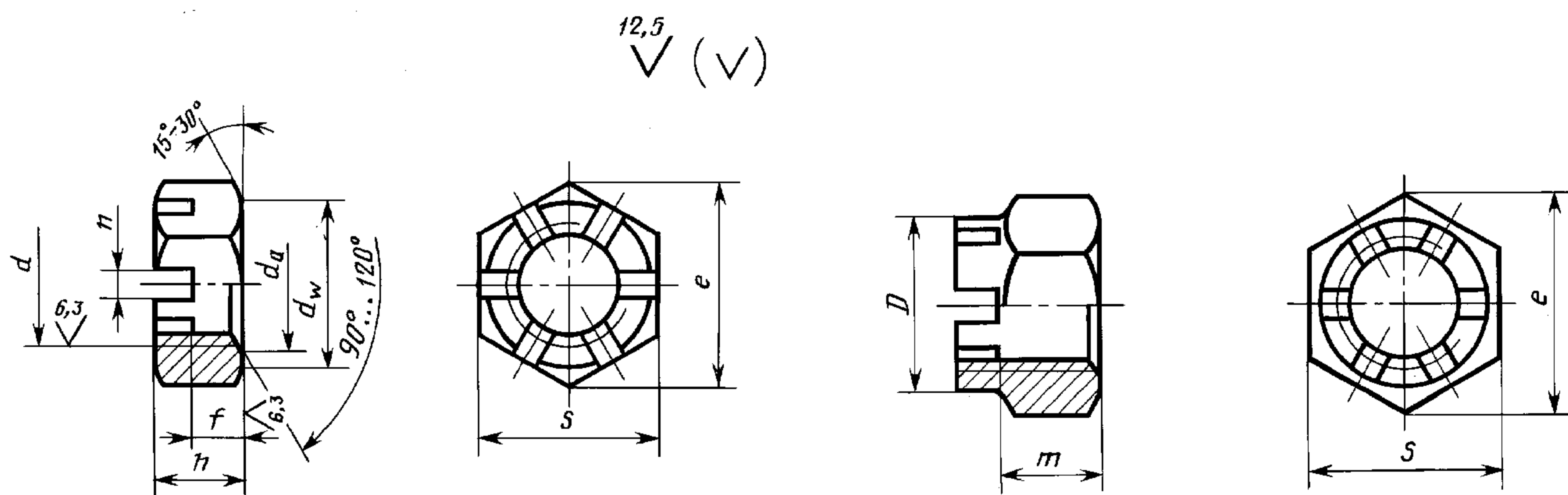
Исполнение 1
