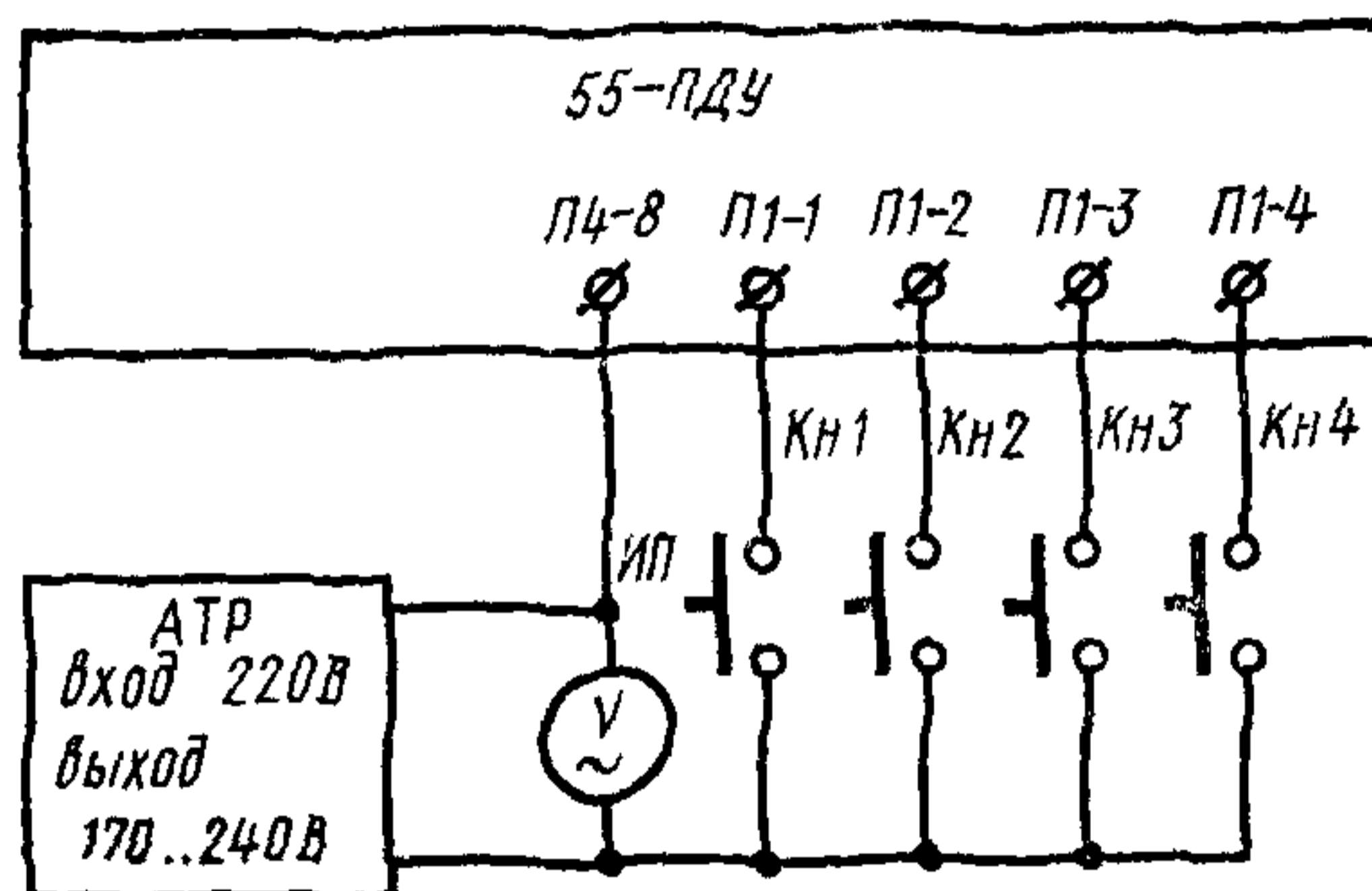
Схема проверки
