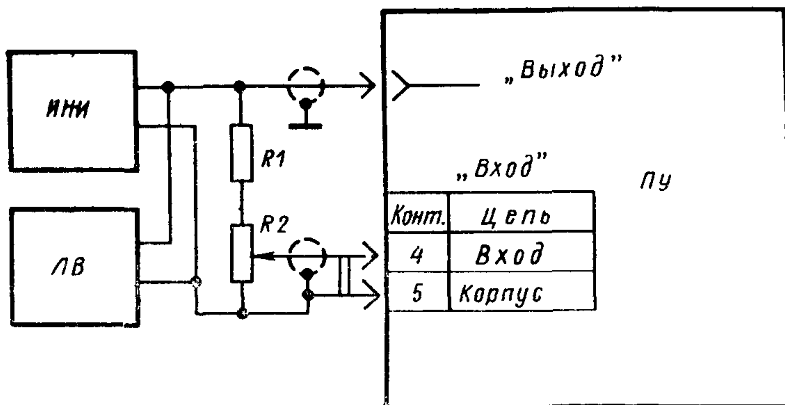
Схема для проверки нелинейных искажений
