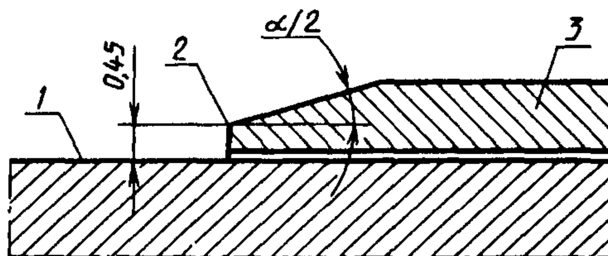
1 — поверхность стебля; 2 — измерительная кромка; 3 — барабан
