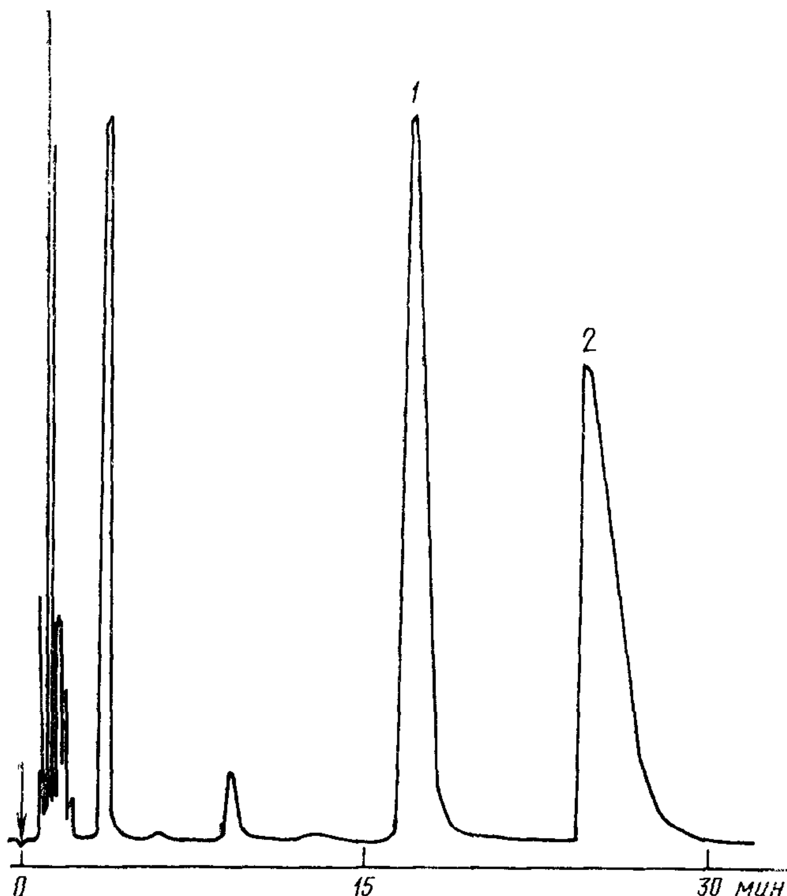
Хроматограмма образца фенхелевого масла
