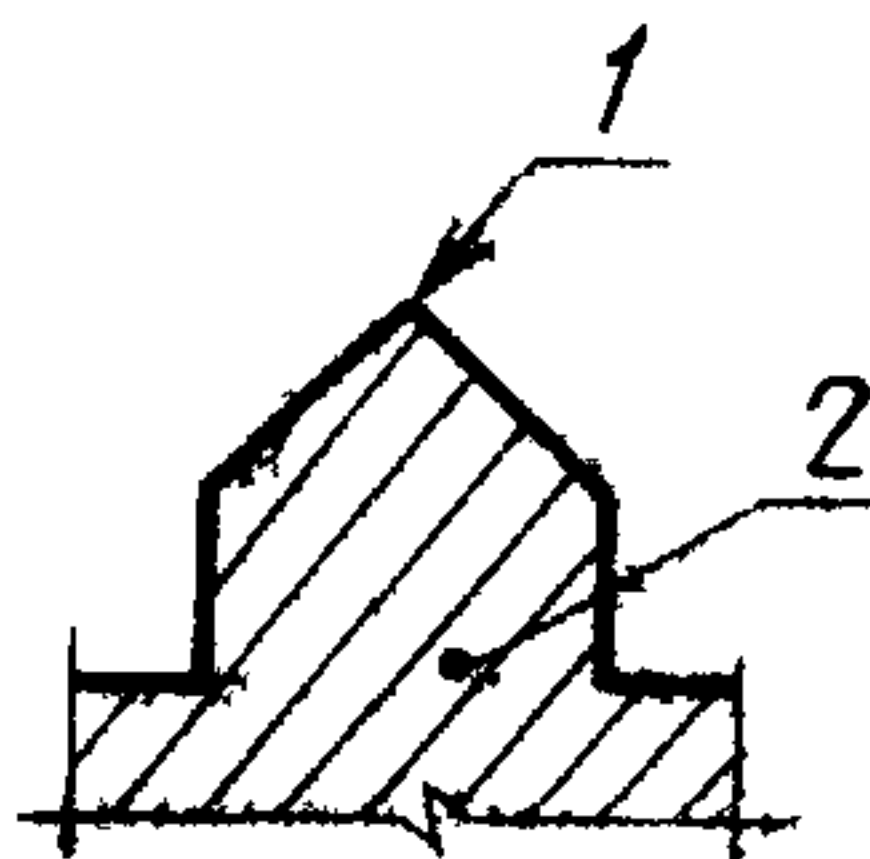
1 — радиус кривизны опоры (макс. 0,25 мм); 2 — опора
