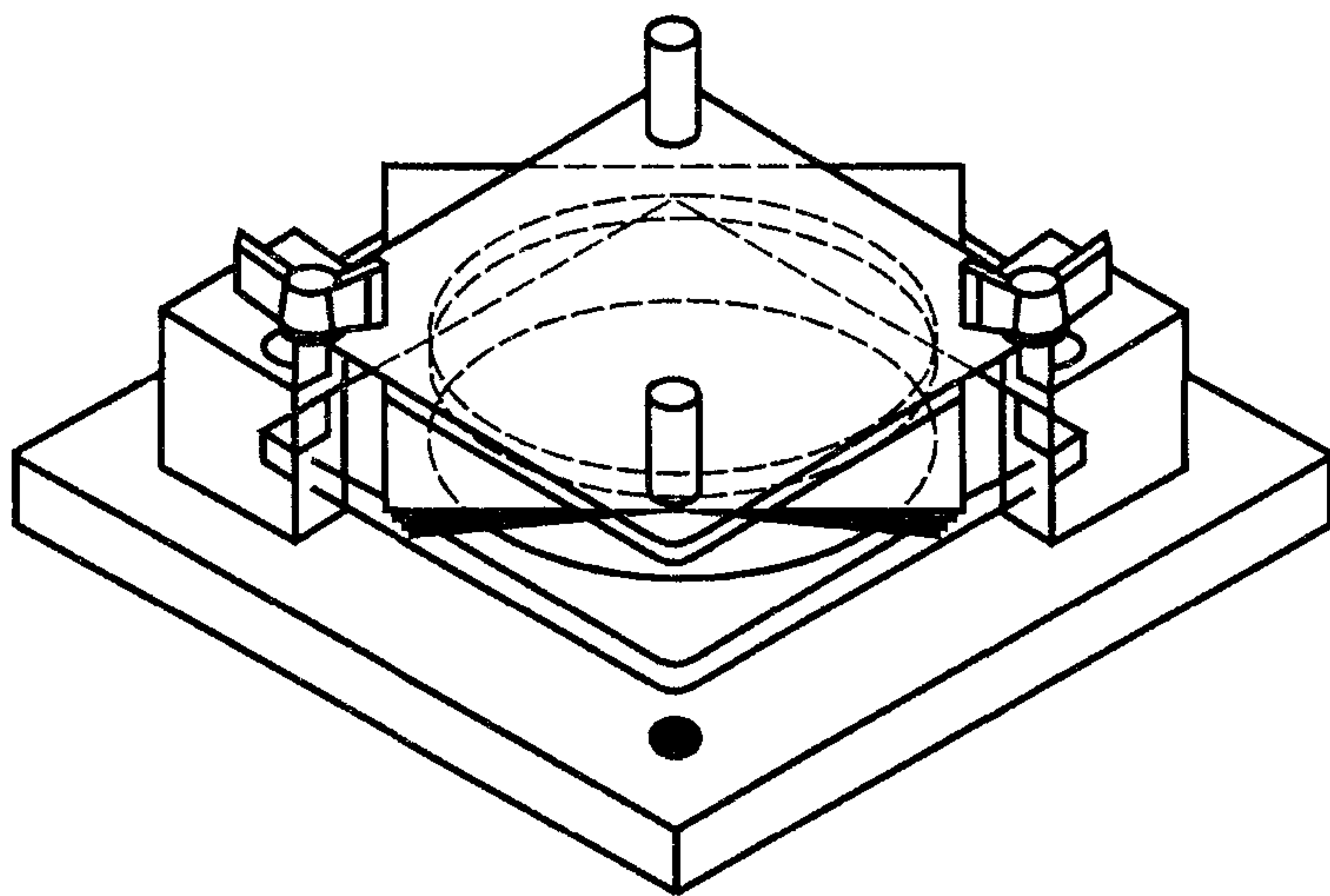
Рисунок 3 — Прибор для определения масловпитываемости бумаги
