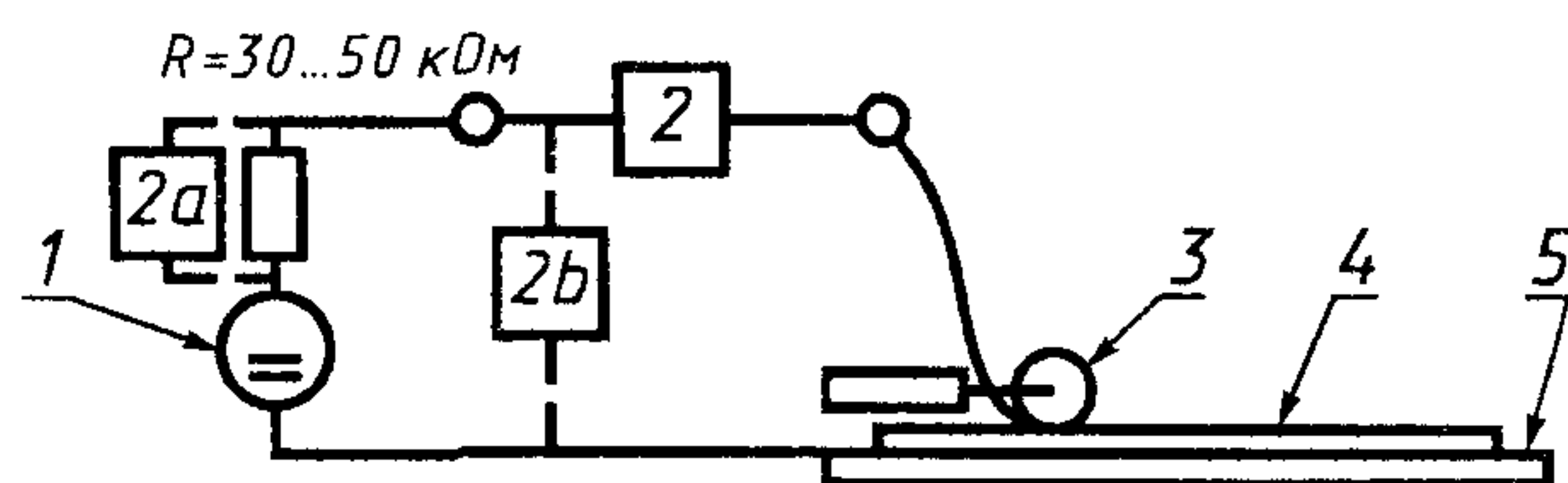
1 — источник напряжения 110 В; 2 — индикаторное и счетное устройство (2a и 2b — возможные расположения); 3 — роликовый электрод; 4 — испытуемый образец; 5 — плоский электрод
