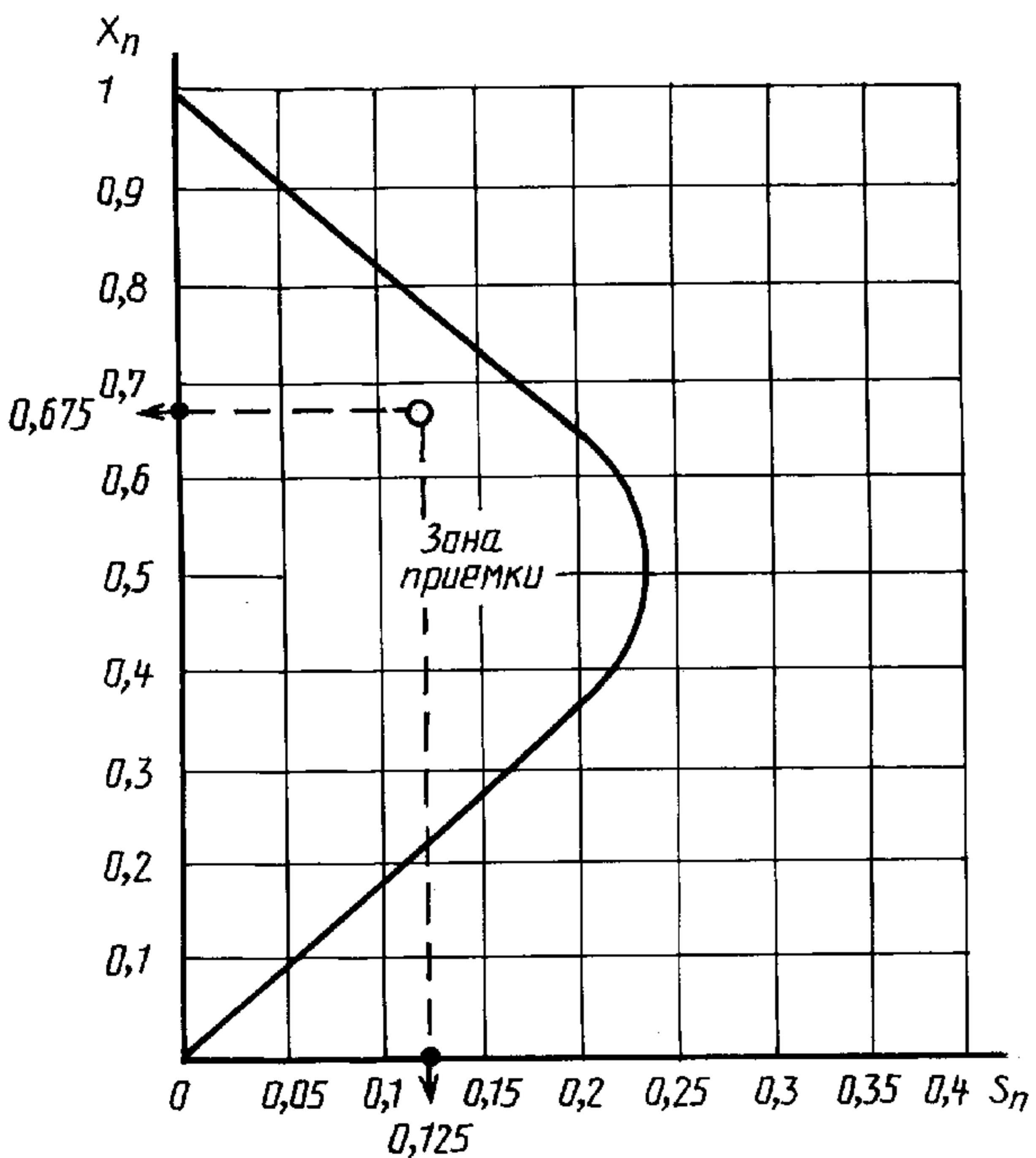
Рисунок 1 — Приемочная кривая для уровня качества AQL=1,5
