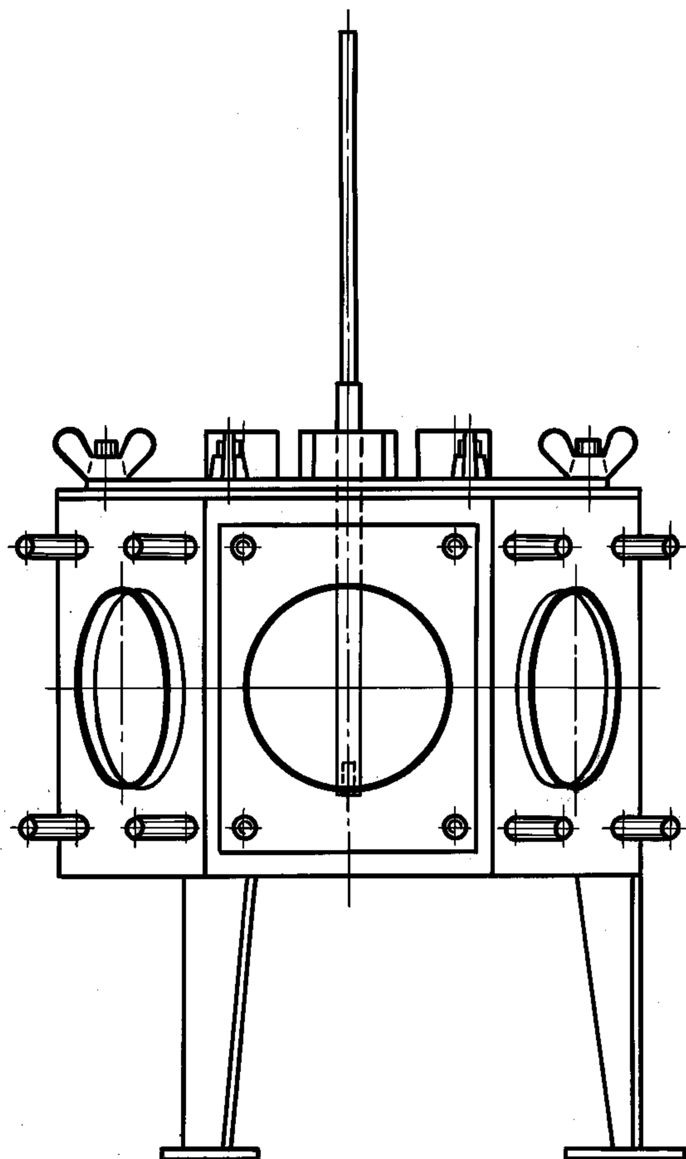
Шестигранный сосуд с крышкой, мешалкой и зажимной пластиной
