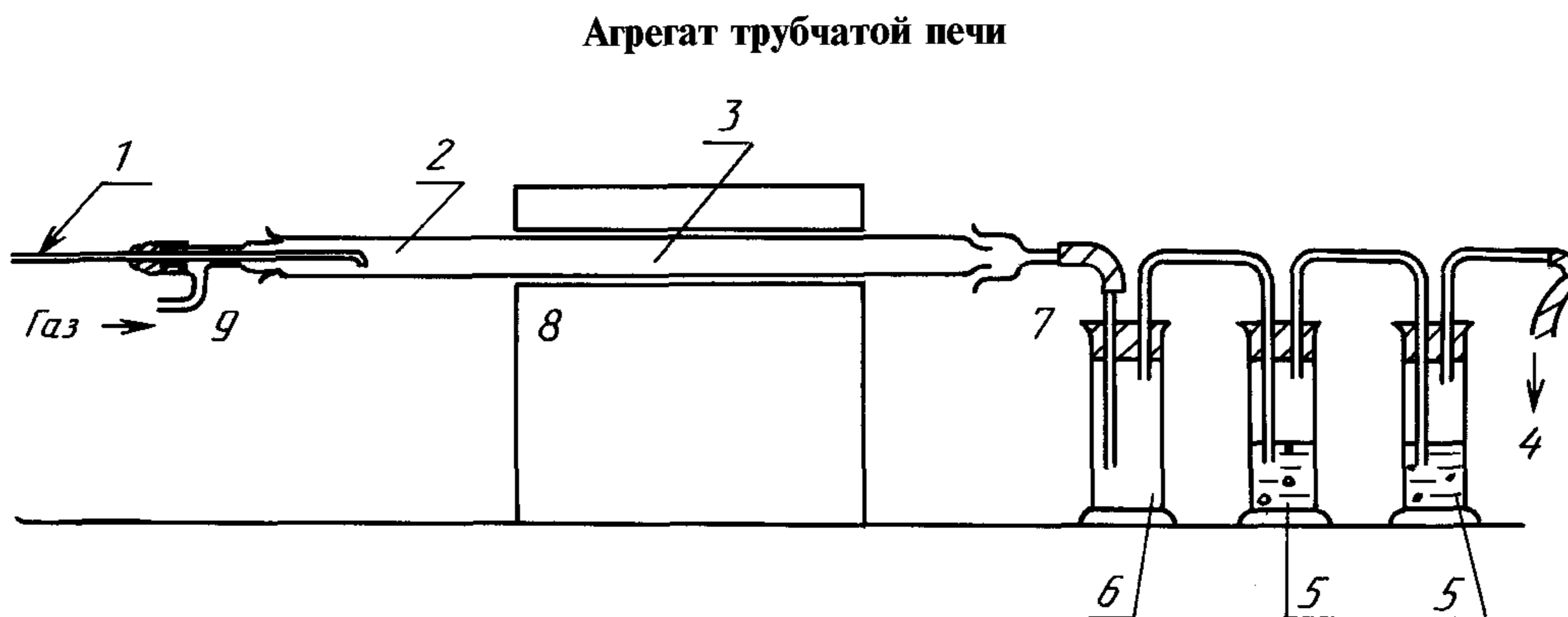
1 — кварцевая палочка с крючком; 2 — охлажденная зона; 3 — центральная горячая зона; 4 — сток; 5 — ловушка с ксилолом; 6 — ловушка для конденсируемых паров; 7 — шлиф 29/32; 8 — трубчатая печь при (850 \pm 25)^\circ\text{C} ; 9 — шлиф 29/32
