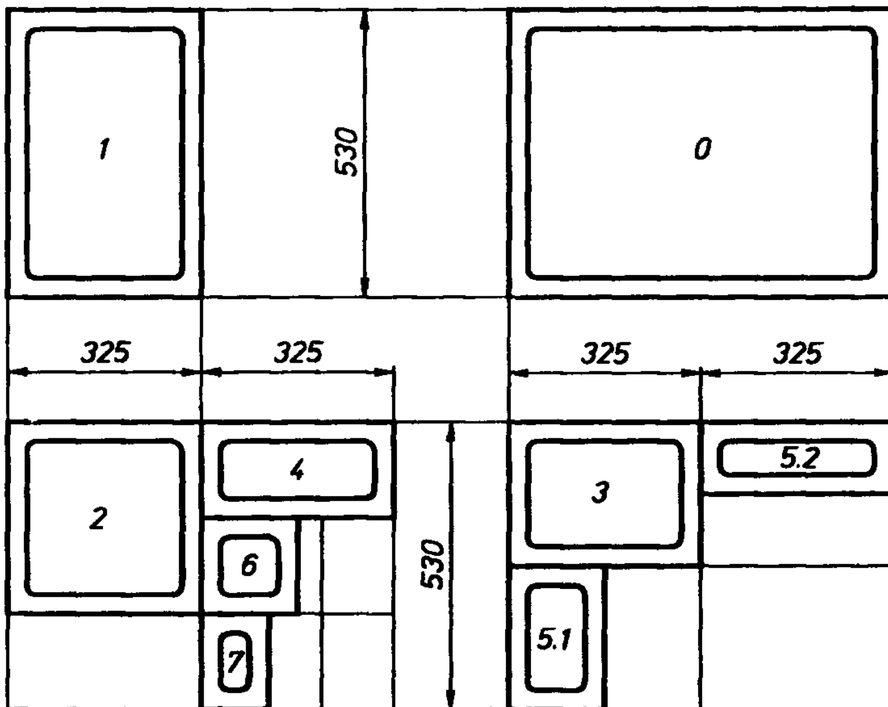
0—7 номера функциональных емкостей Рисунок 1
