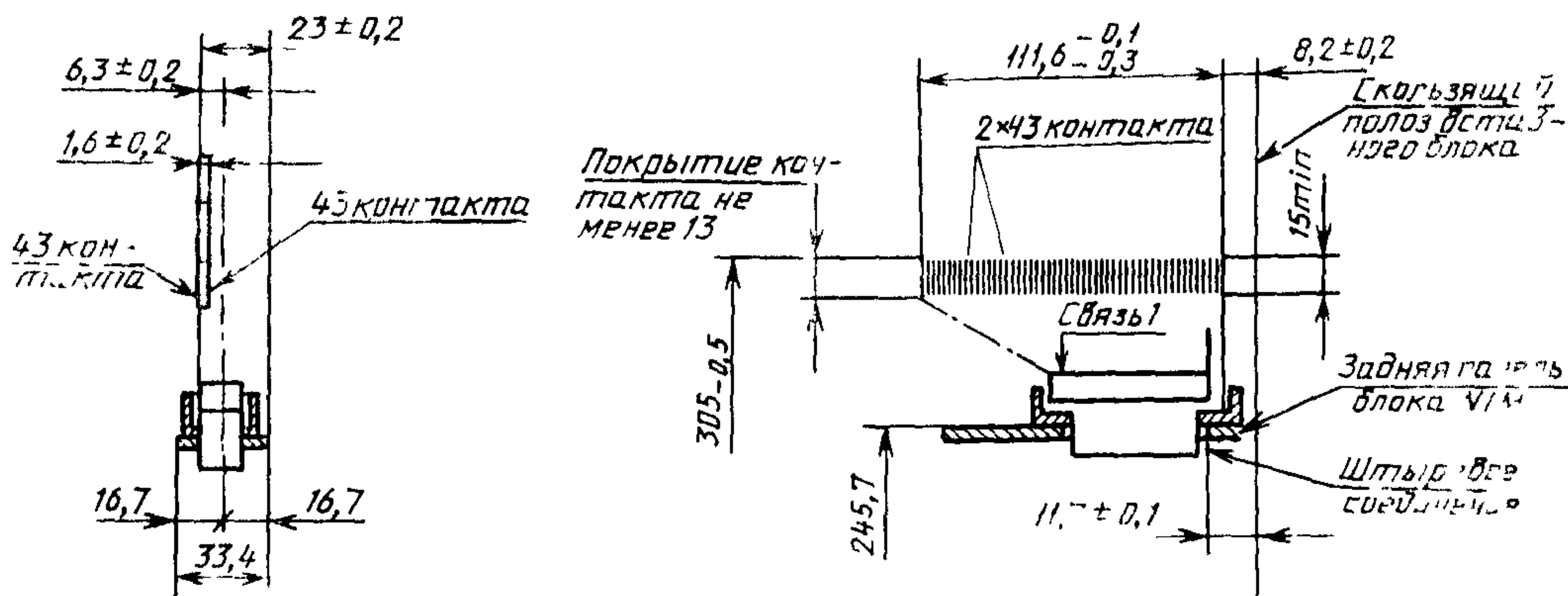
Рисунок 6 — Вентилируемый край. Вид спереди
