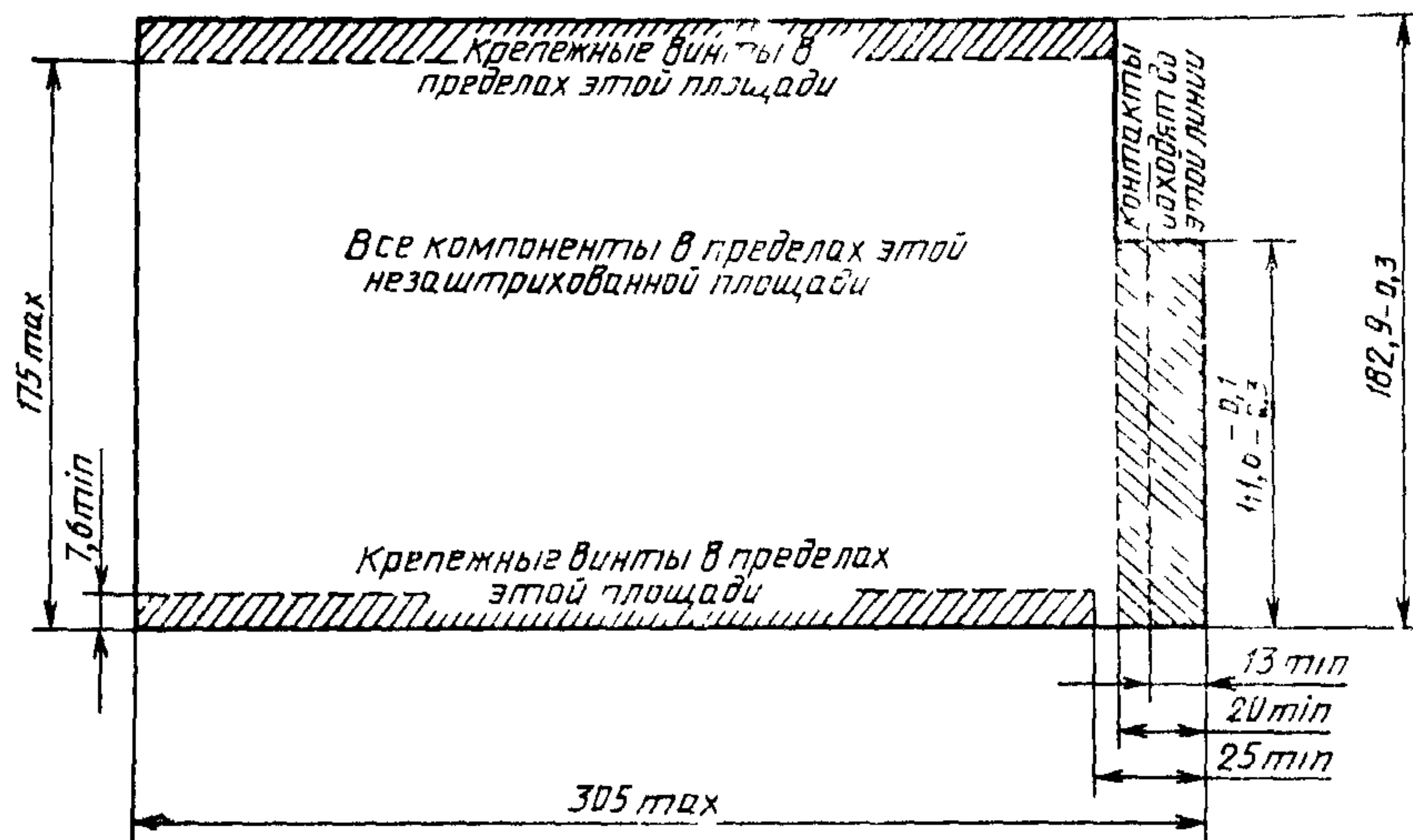
Рисунок 8 — Типовая печатная плата
