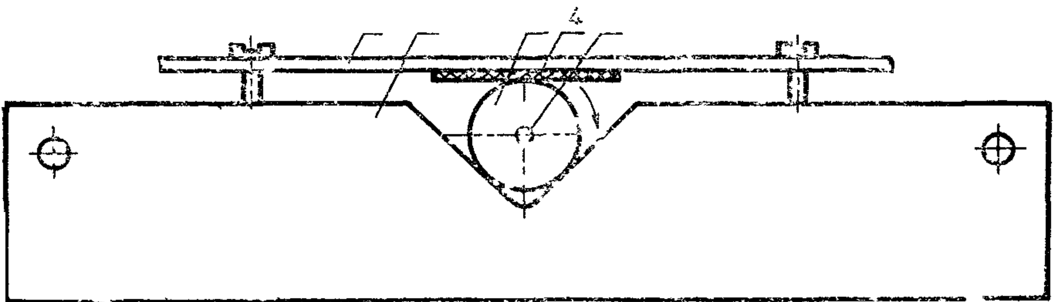
1 — прижим; 2 — призма; 3 — наконечник; 4 — прокладка, 5 — сердцевина волокна
