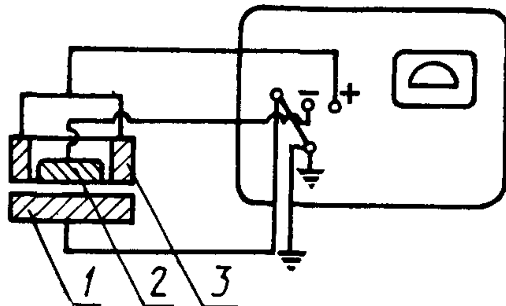
1—охранный электрод; 2—измерительный электрод; 3—высоковольтный электрод
