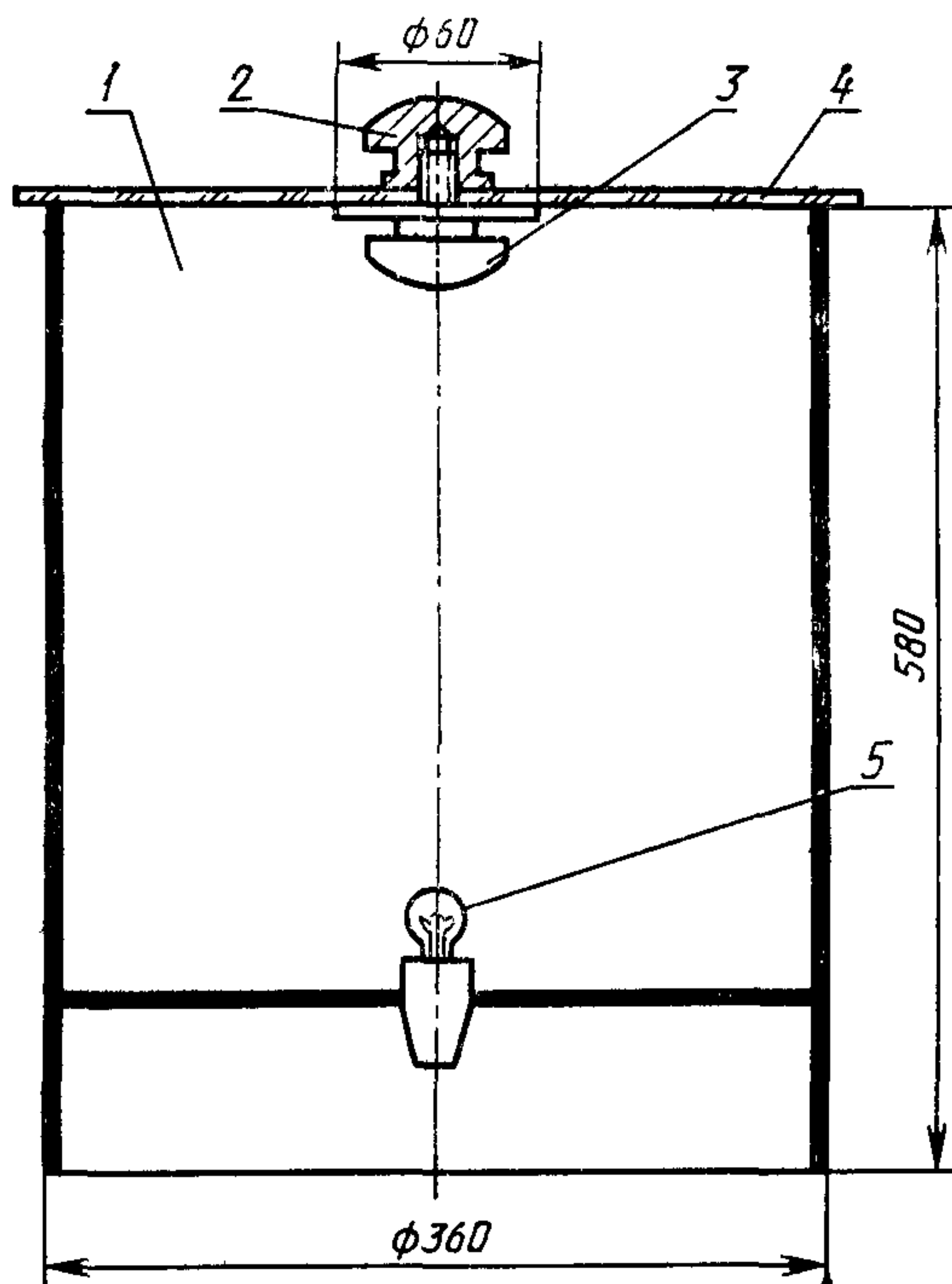
1—корпус; 2—ручка; 3—винт; 4—крышка; 5—источник освещения
