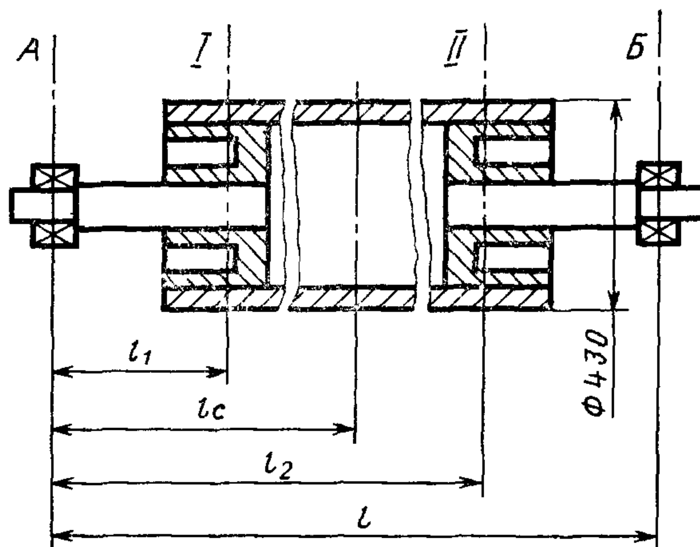
Схема расположения плоскостей коррекции вала
