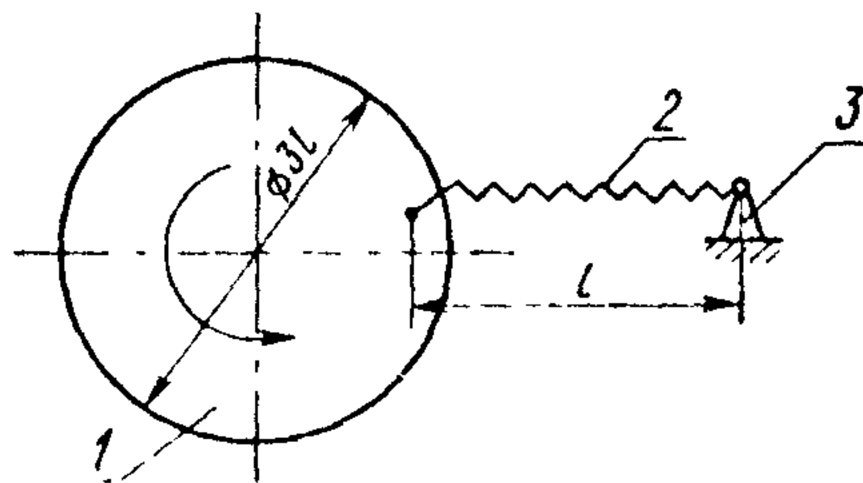
1 — диск; 2 — спиральный шнур; 3 — крепление
