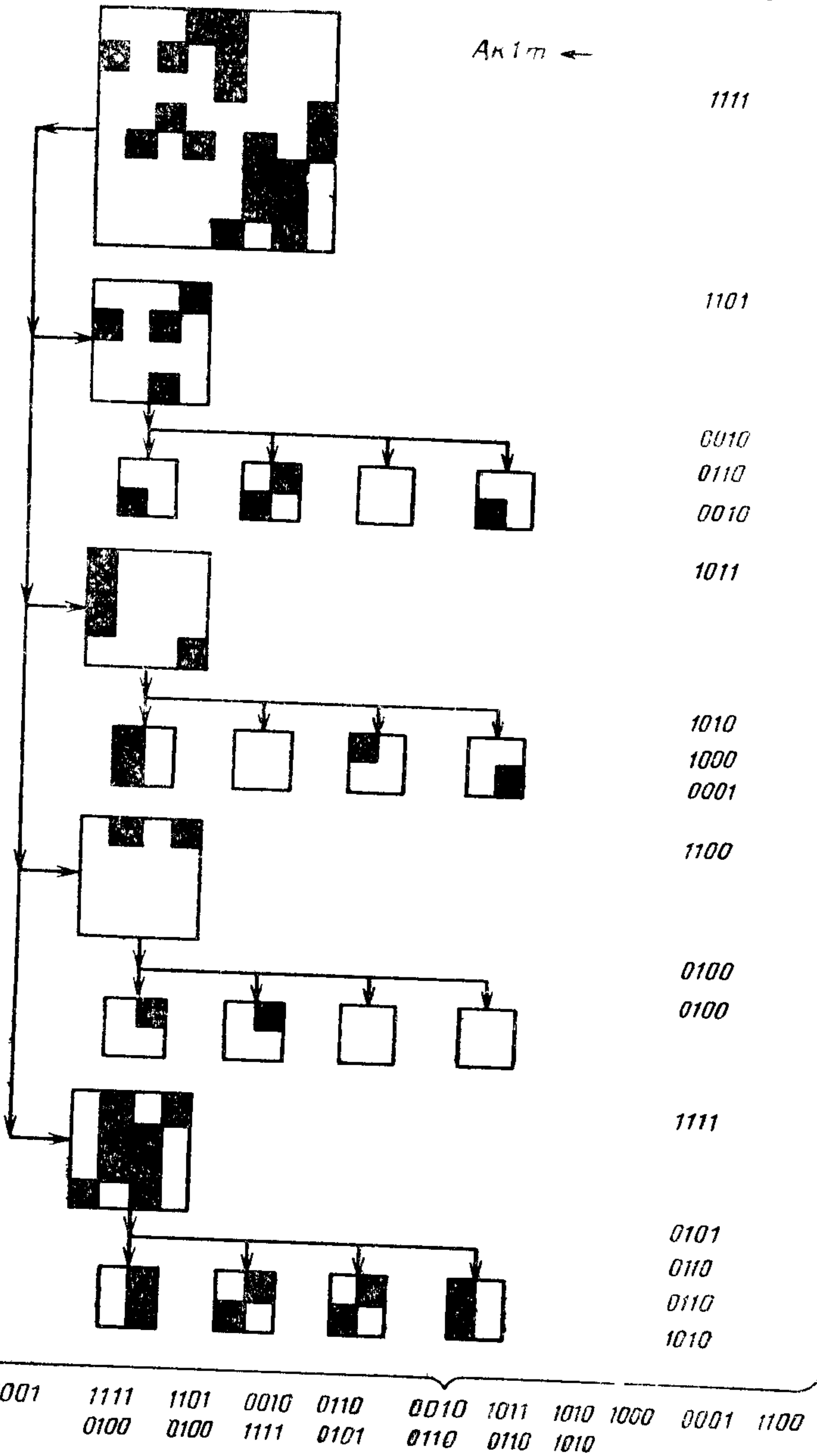
Пример кодирования небелого квадрата A_{k1m} с контуром, выделенным в направлении строк справа налево
