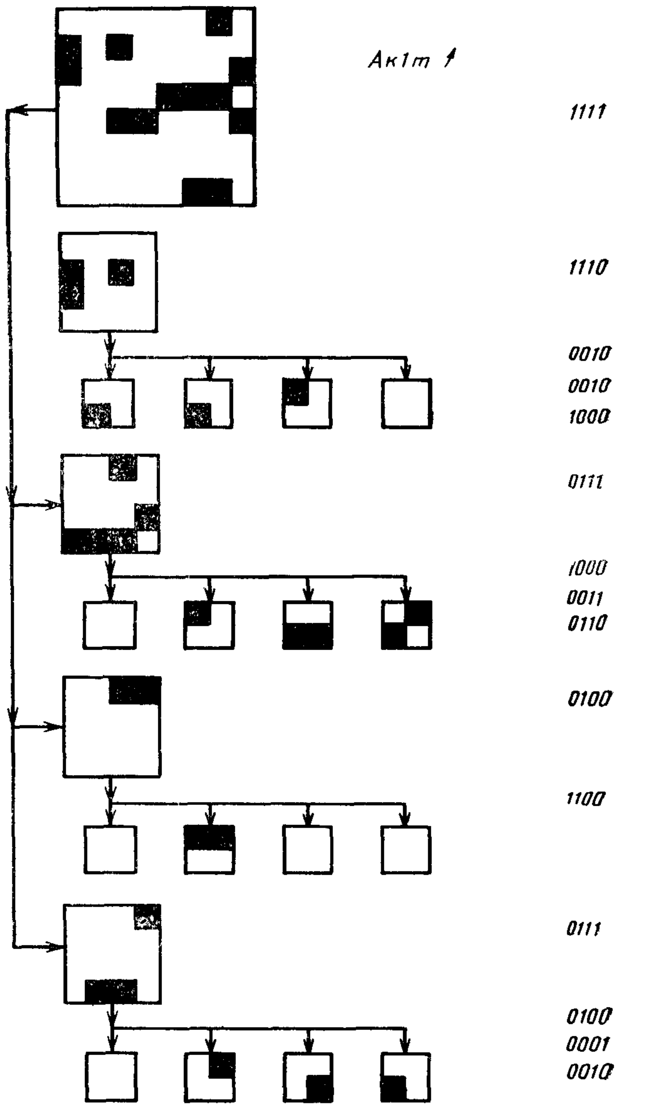
Пример кодирования небелого квадрата A_{k1m} с контуром, выделенным в направлении столбцов снизу вверх
