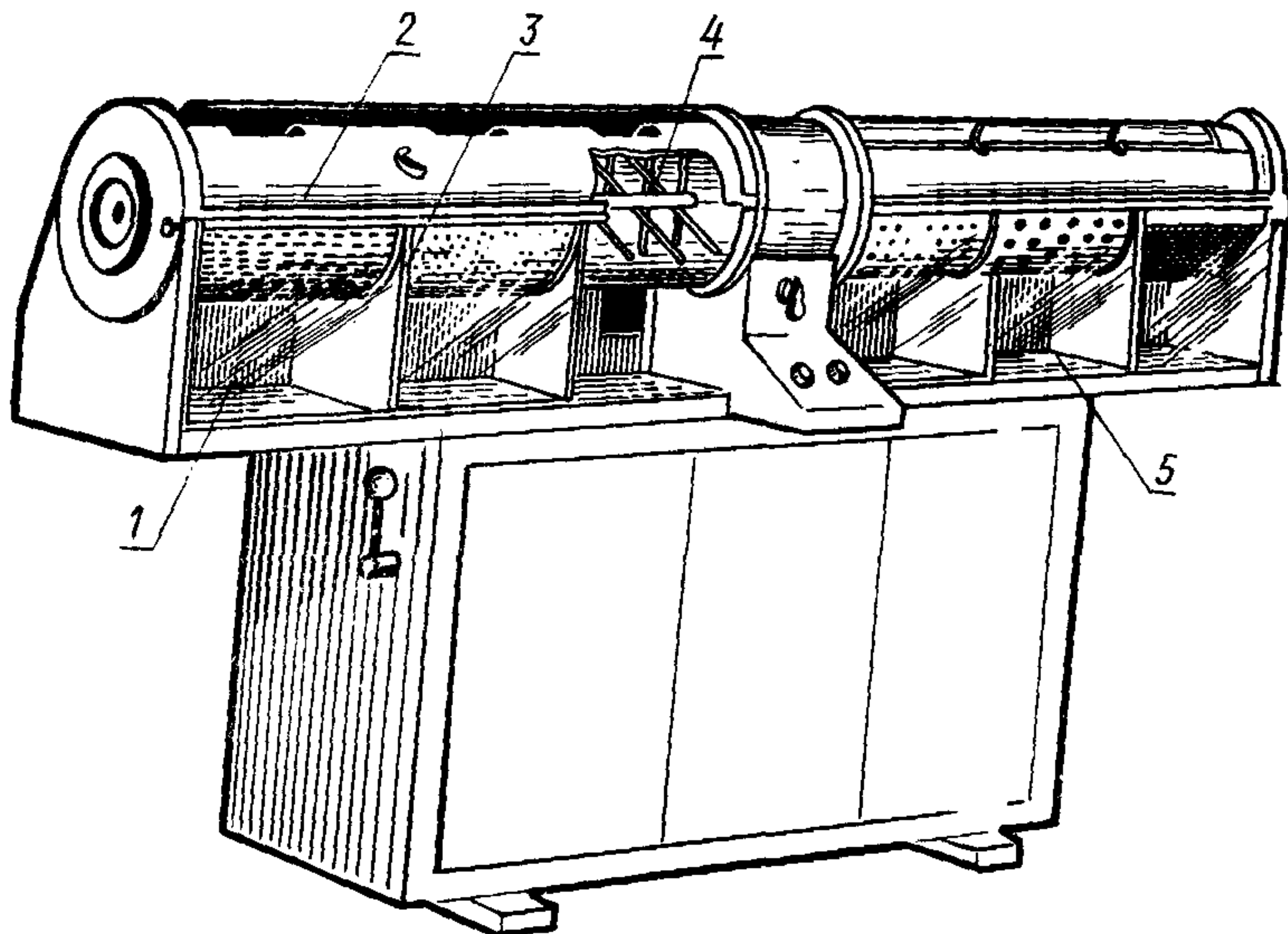
1 — рабочая камера; 2 — загрузочная воронка; 3 — перегородка; 4 — вал с колками; 5 — сетка
