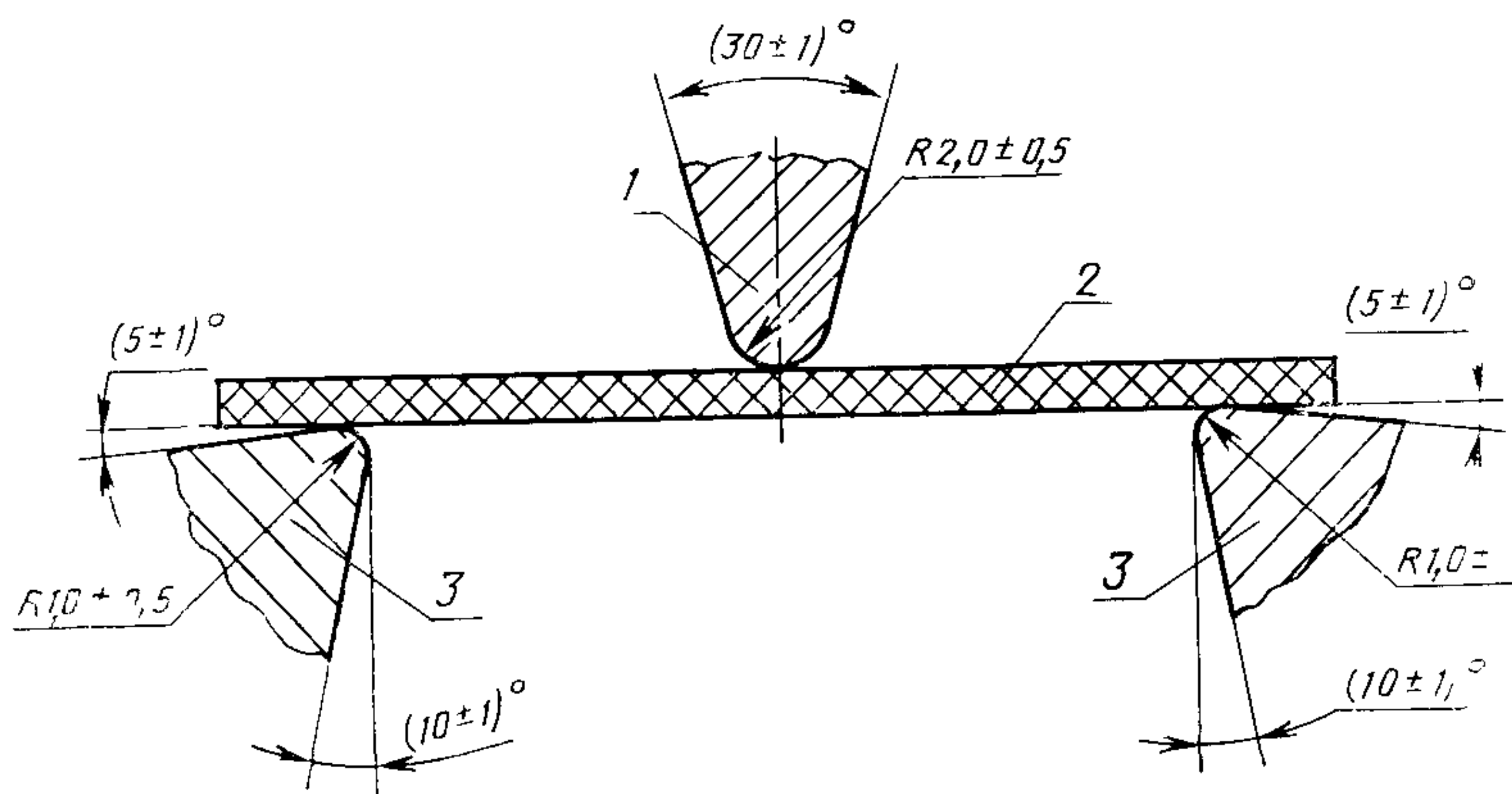
1—боек маятника, 2—образец 3—опоры
