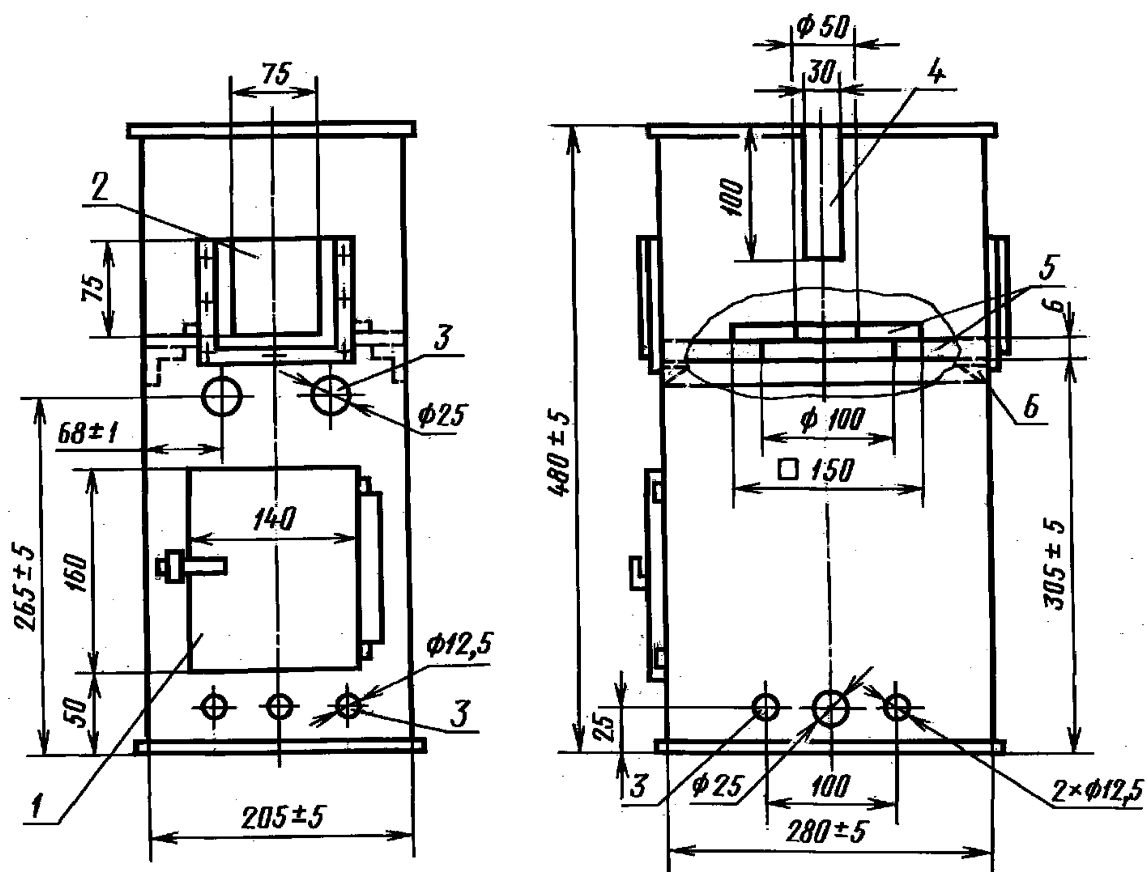
1 — дверца; 2 — окошко; 3 — отверстия; 4 — прорезь; 5 — асбестовые пластинки; 6 — опора
