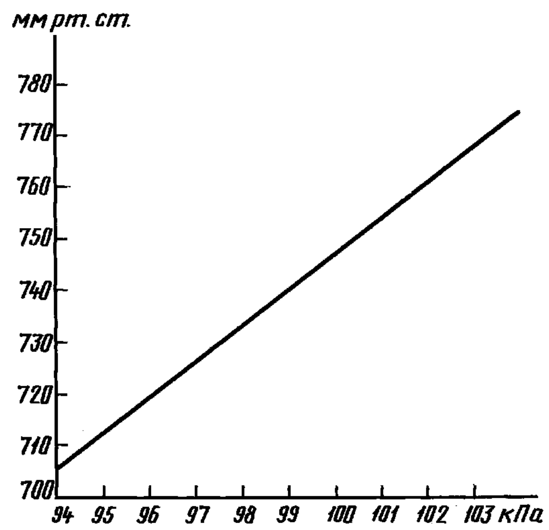
Диаграмма соотношения единиц измерения атмосферного давления
