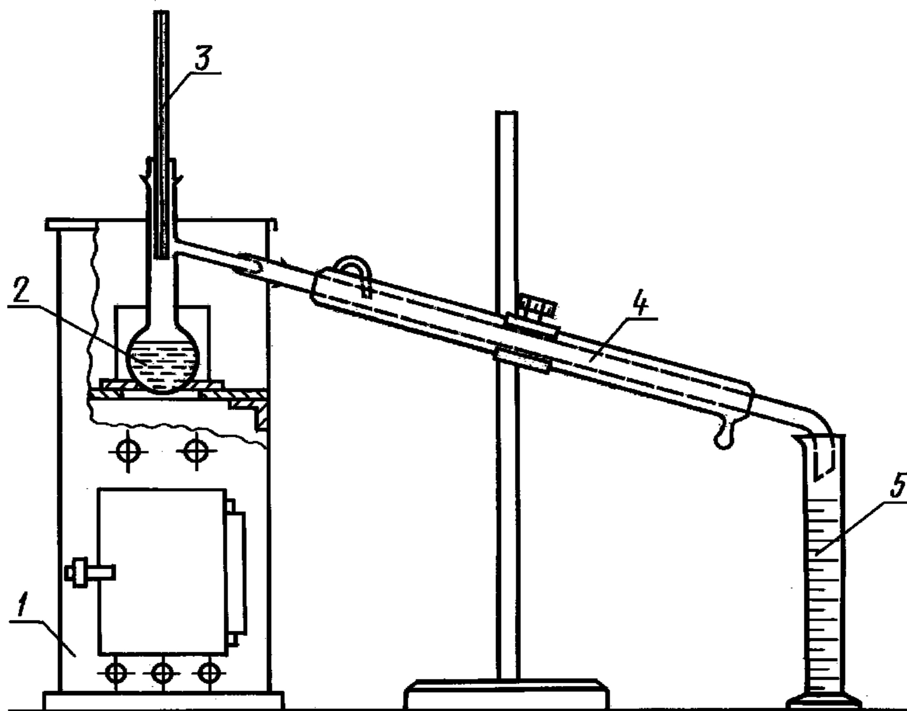
1 — кожух; 2 — перегонная колба; 3 — измерительный термометр; 4 — холодильник; 5 — цилиндр-приемник
