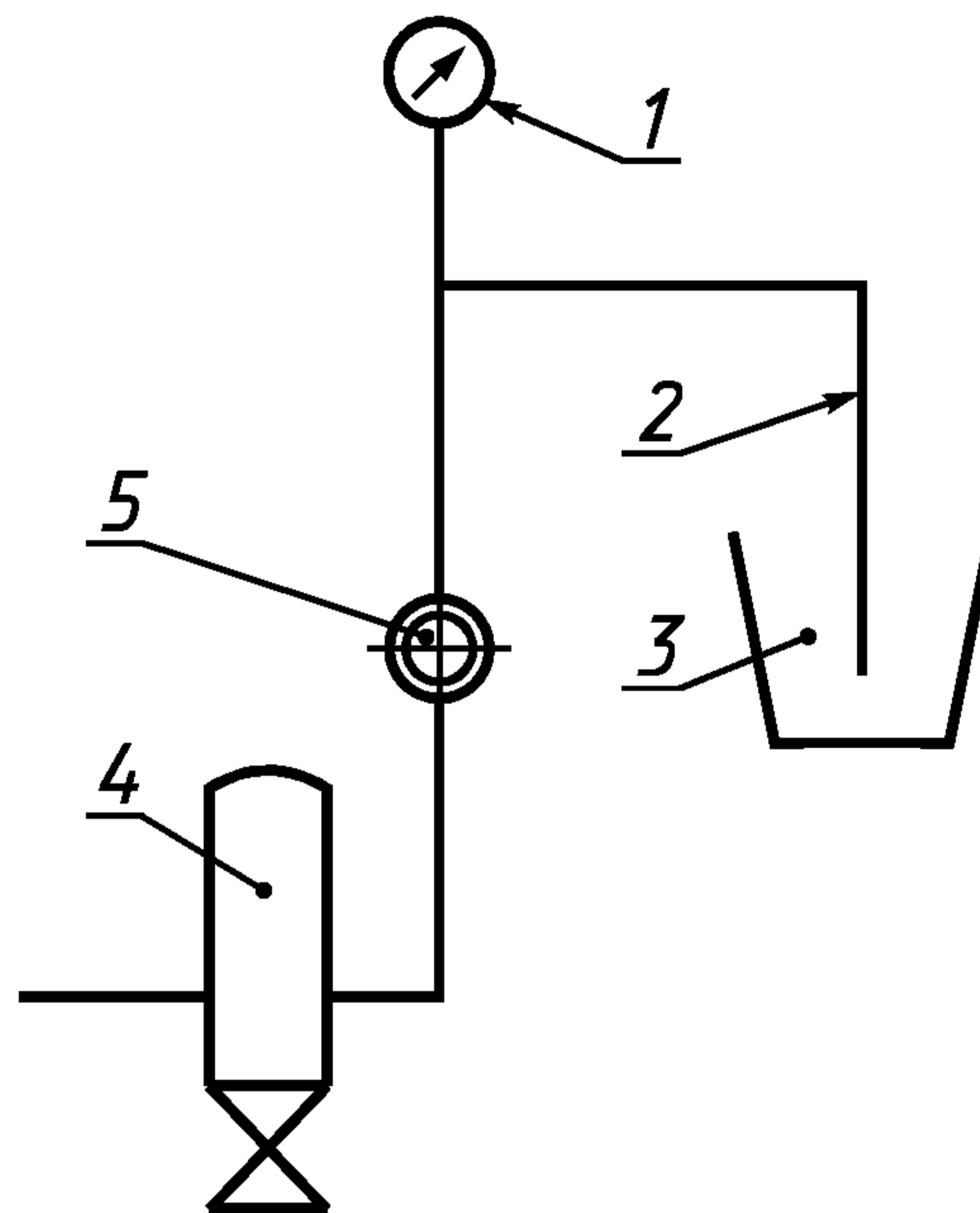
Схема устройства аппарата
