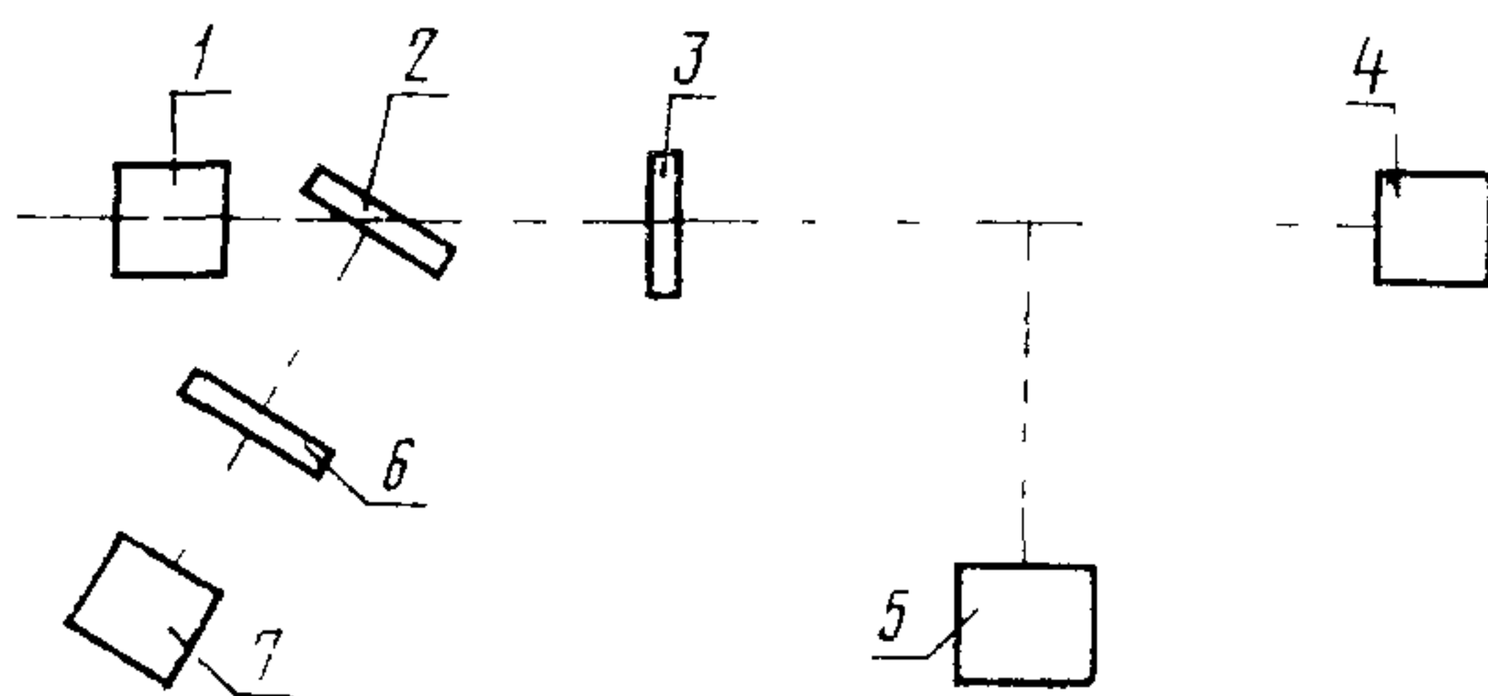
Блок-схема установки для определения чувствительности измерительных приборов
