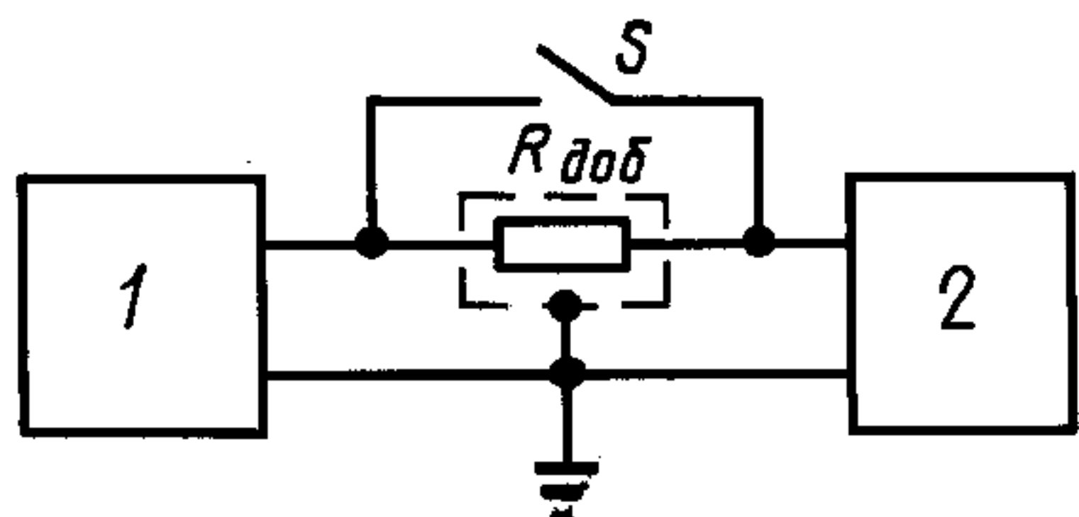
Схема определения входного сопротивления
