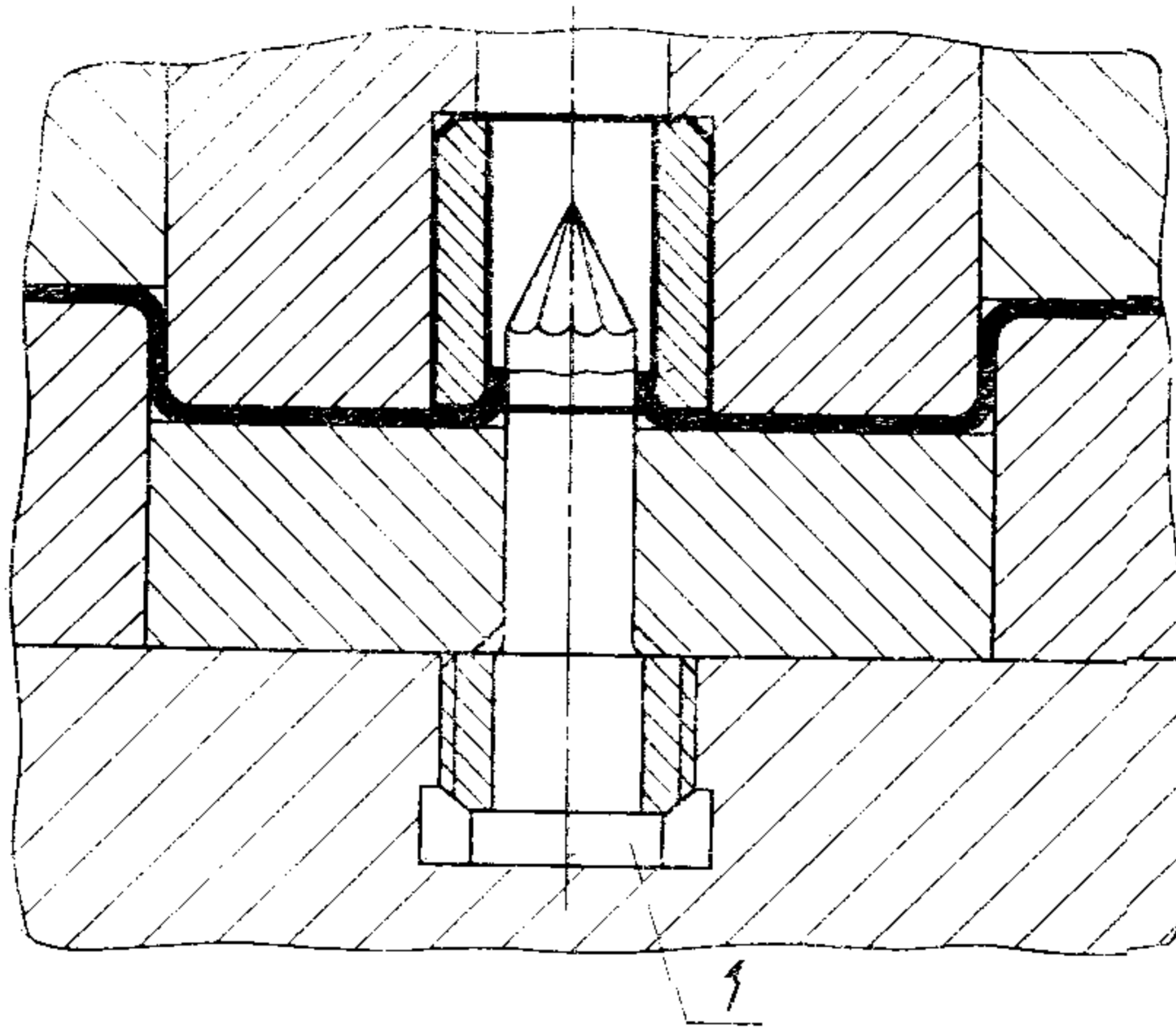
I —проколочный пуансон по ГОСТ 24533—80
